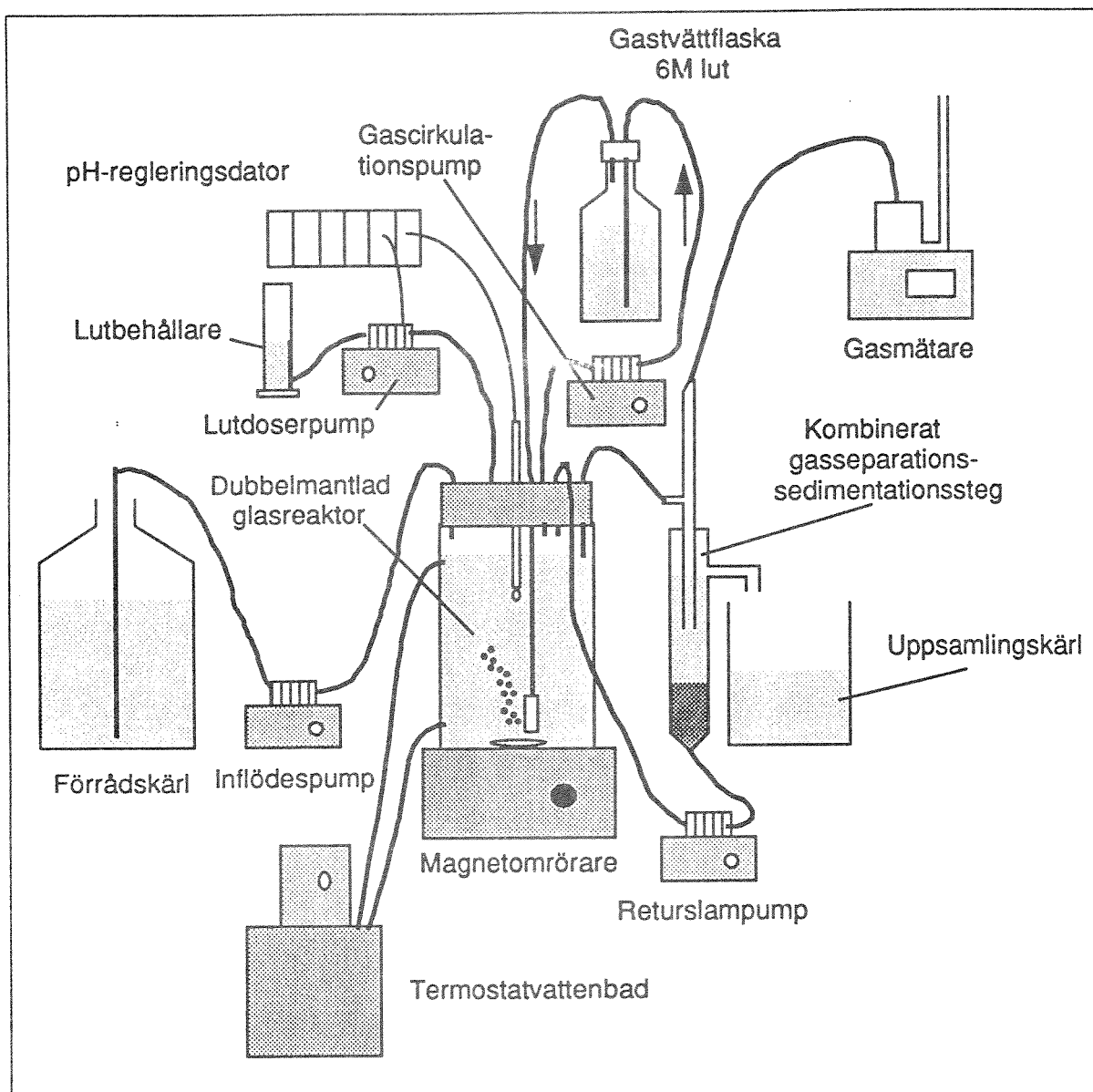
Figur 2. Kontaktprocess i labskala använd i de kontinuerliga försöken. Avloppsvattnet pumpades från ett förrådskärl till den dubbelmantlade glasreaktor, varifrån det fick gå vidare till ett kombinerat gasseparations/sedimentationssteg tillsammans med i reaktorn bildad biogas. I separationssteget avskiljdes först gasen som fick gå ut via en gasmätare. Slammet i utgående vatten fick därefter sedimentera för återföring till reaktorn via en returslampump, medan klarfasen fick bräddas ut till ett uppsamlingskärl. Temperaturen i reaktorn hölls konstant vid 37°C genom cirkulation av tempererat vatten från ett termostatvattenbad genom den yttre manteln på reaktorn och pH upprätthölls vid 7.0 genom kontinuerlig pH-mätning och automatisk titrering med 1M NaOH m.h.a. en dator och en lutdoserpump. För att undvika att bildat svavelväte skulle förgifta processen cirkulerades gasfasen i reaktorn kontinuerligt genom en gastvättflaska innehållande 6M NaOH i vilken huvuddelen av den bildade sulfiden absorberades.
