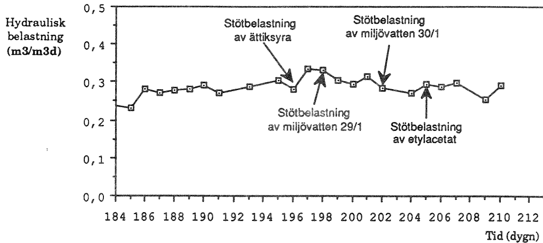
Figur 35. Hydraulisk belastning plottad mot tiden för reaktor 4 under försöksperiod med stöbelastningar av olika komponenter.
