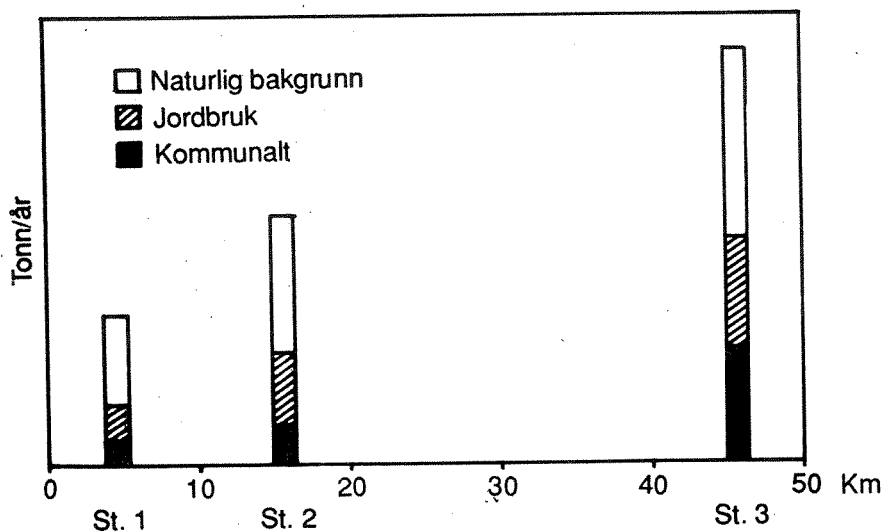
Fig. 8.7 Stofftransport i et vassdrag fordelt på kilder. Andelen kan også fremstilles som prosent. (Avstand i km fra referansepunkt.)
