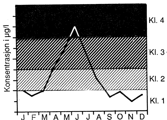
Fig. 8.3 Elvestasjon. Fremstilling av konsentrasjonsverdiene av et stoff ved månedlige observasjoner gjennom et år. Observasjonens klasseverdi (forurensningsgrad) skal fremgå.
