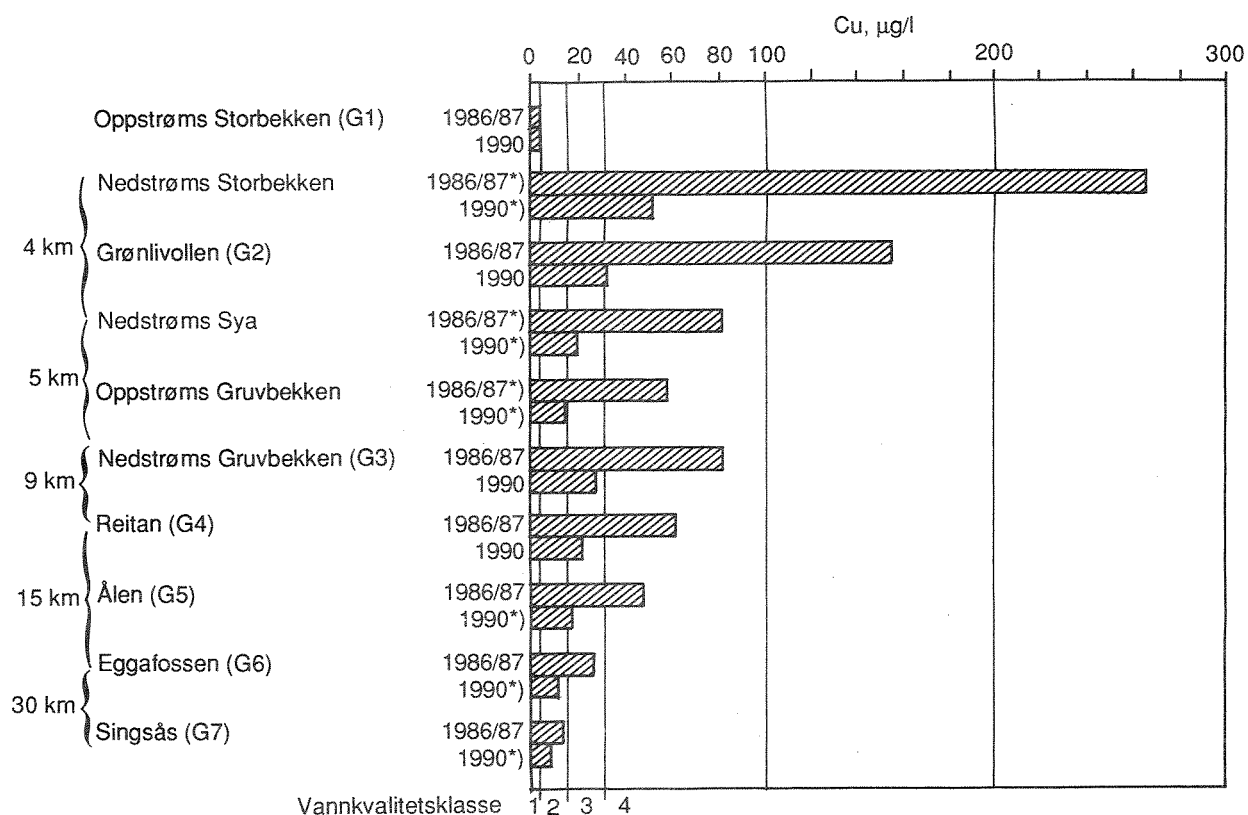
Figur 5. Middelerverdier av kobberkonsentrasjoner i øvre deler av Gaula for perioden juni t.o.m. desember i 1986/87 og 1990. Verdier merket med stjerne *) er beregnet ut fra teoretisk fortykning fra stasjoner med målte verdier. For bakgrunnsstasjonen oppstrøms Storbekken (G1) er det regnet med uendrede forhold etter 1986/87. Lengden på elvestrekninger er angitt. Det er gode muligheter for å etablere fiskebestander fra 20 µg Cu/l og lavere. Vannkvalitetsklassene er etter SFT 1989.
