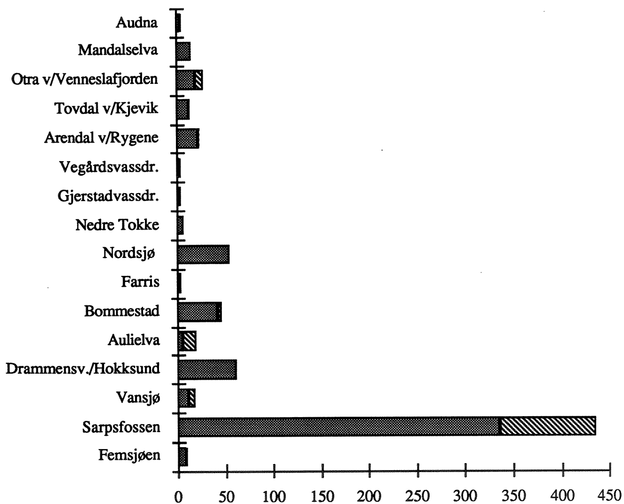
Figur 18. Nødvendige reduksjoner i tilførsler av fosfor for å nå anbefalte krav til vannkvalitet (skravert areal). Hel søyle angir dagens tilførsler ( det grå pluss det skraverte arealet).
