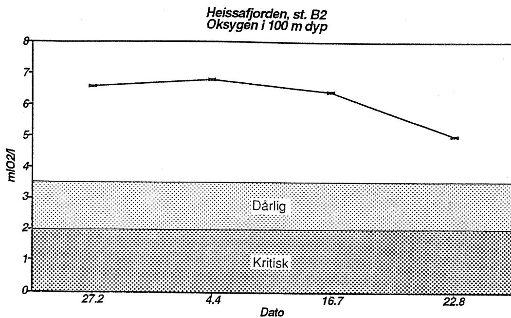
Fig. 5.13 Oksygenmålinger i 100 m dyp i Heissafjorden (st. B2) i 1990.
