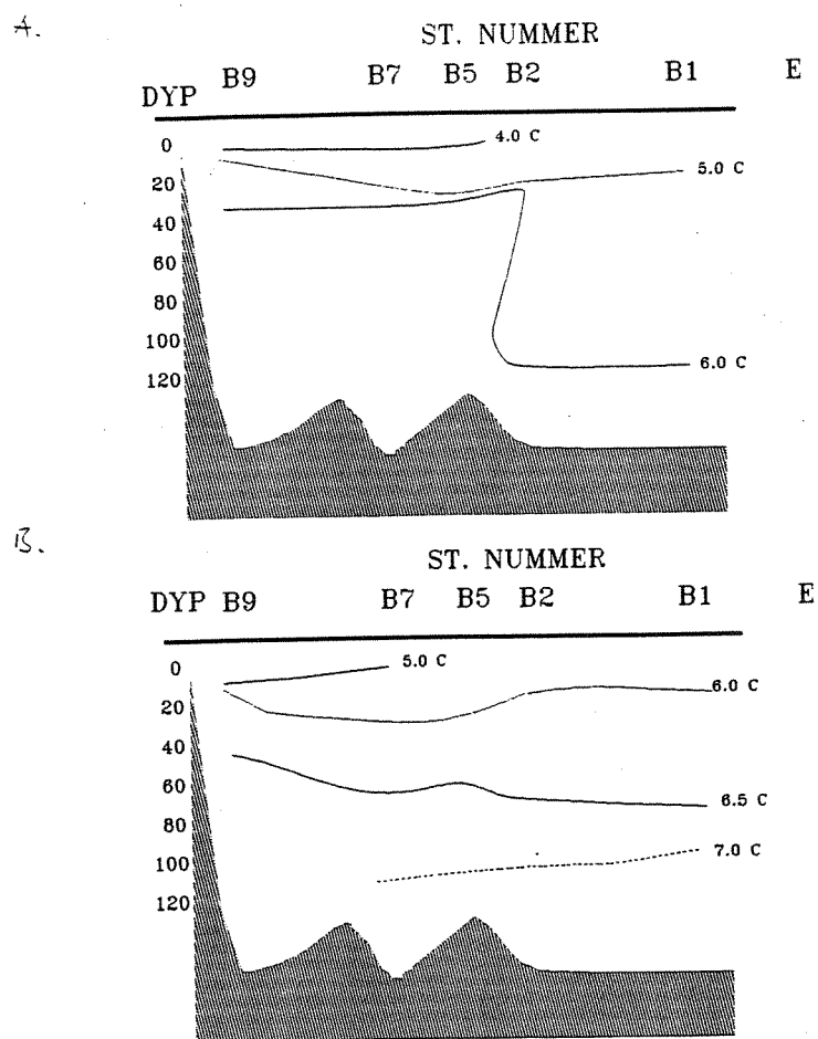
Fig. 9.4 Hydrografisk snitt for 13. mars og 4. april.
