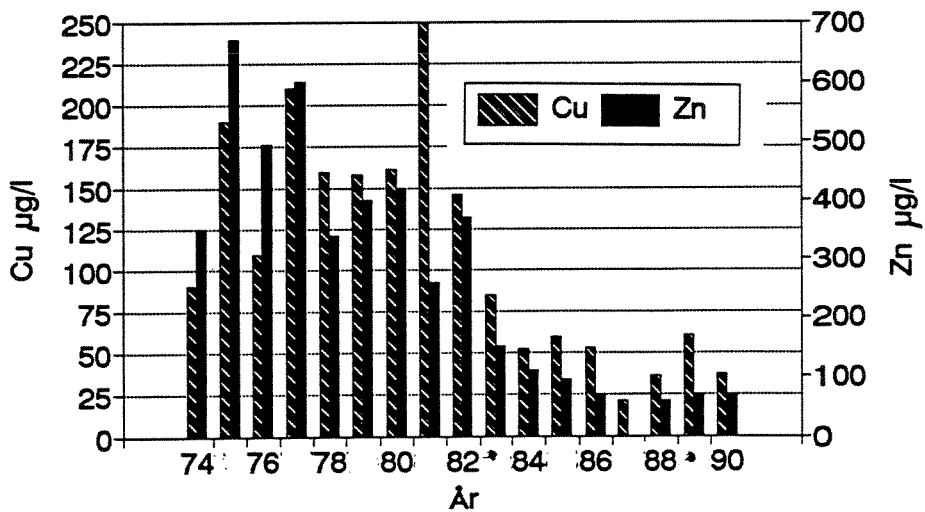
Fig.5C Orkla ved Vormstad 1974-90 Maks.verdier Cu og Zn
