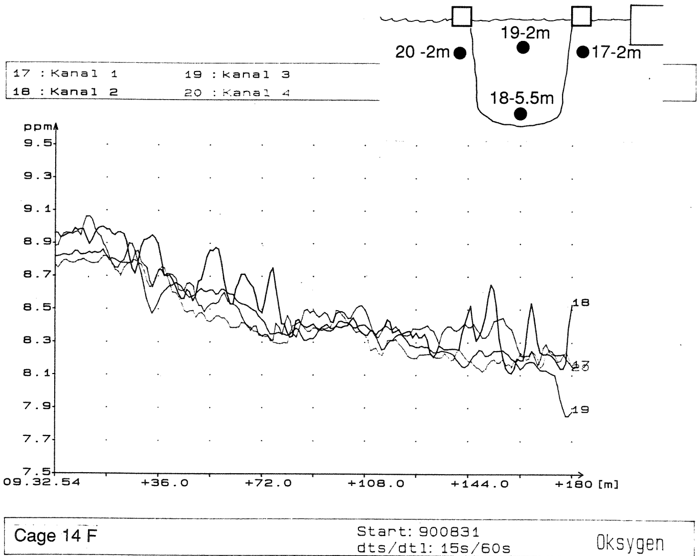
Figur 6 Variasjon i oksygeninnhold på innsiden og utsiden av merd 14 F, Akvaprodukt A/S
