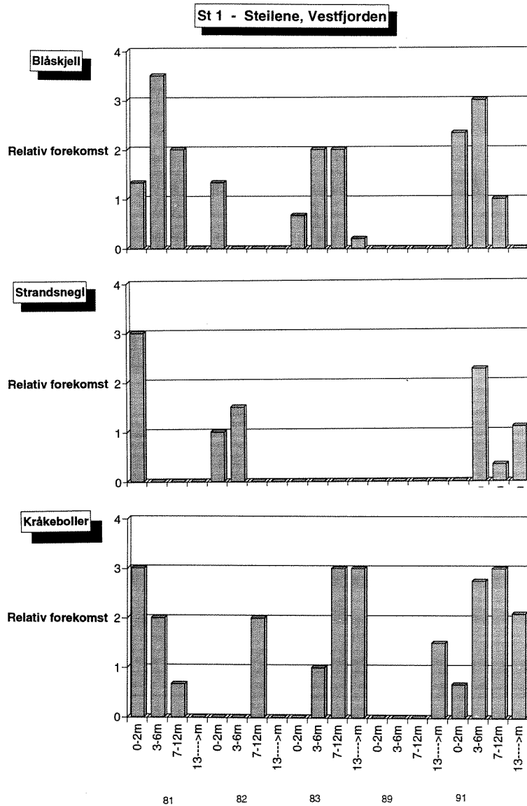
Fig. 33. Relativ forekomst av blåskjell, strandsnegl og kråkeboller på Steilene fra 1981 til 1991 i forskjellige dypintervall.
