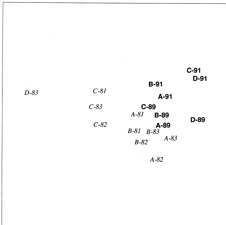
Vedleggsfigur 6. Dendrogram og MDS-plot over algevegetasjonen på st.6 Nakkholmen, fra 1981 til 1991.
