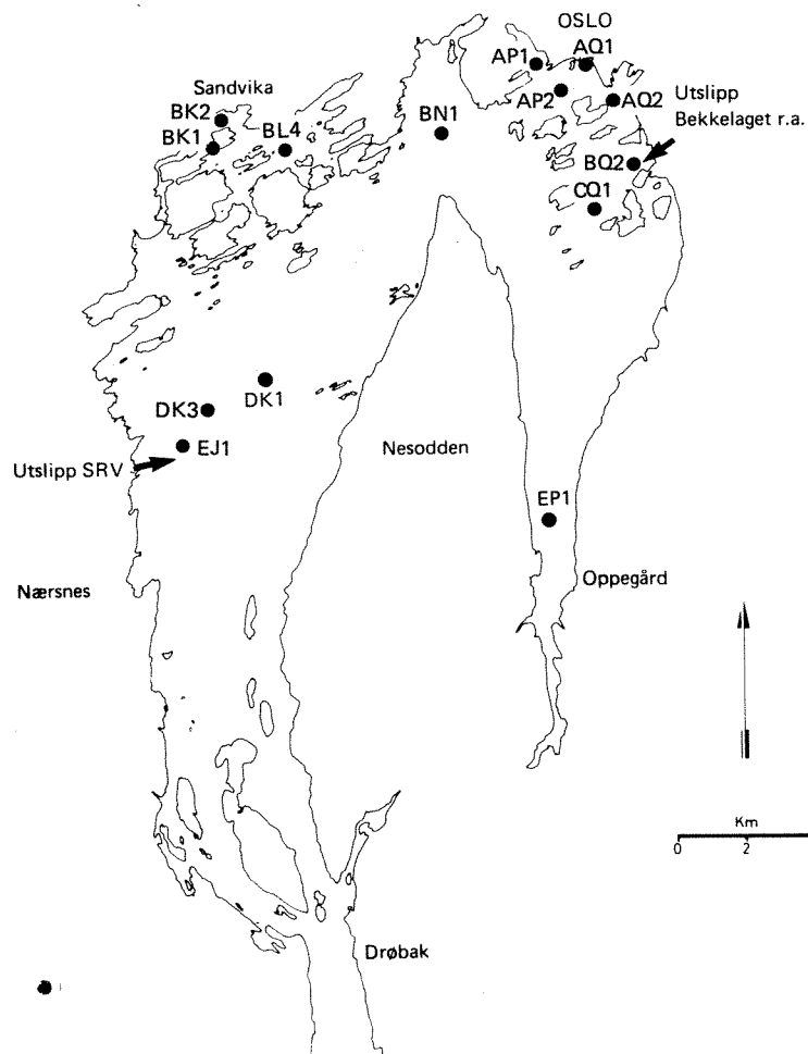
Figur 4. Stasjonsnett for overflateobservasjoner, juni-august 1991.
