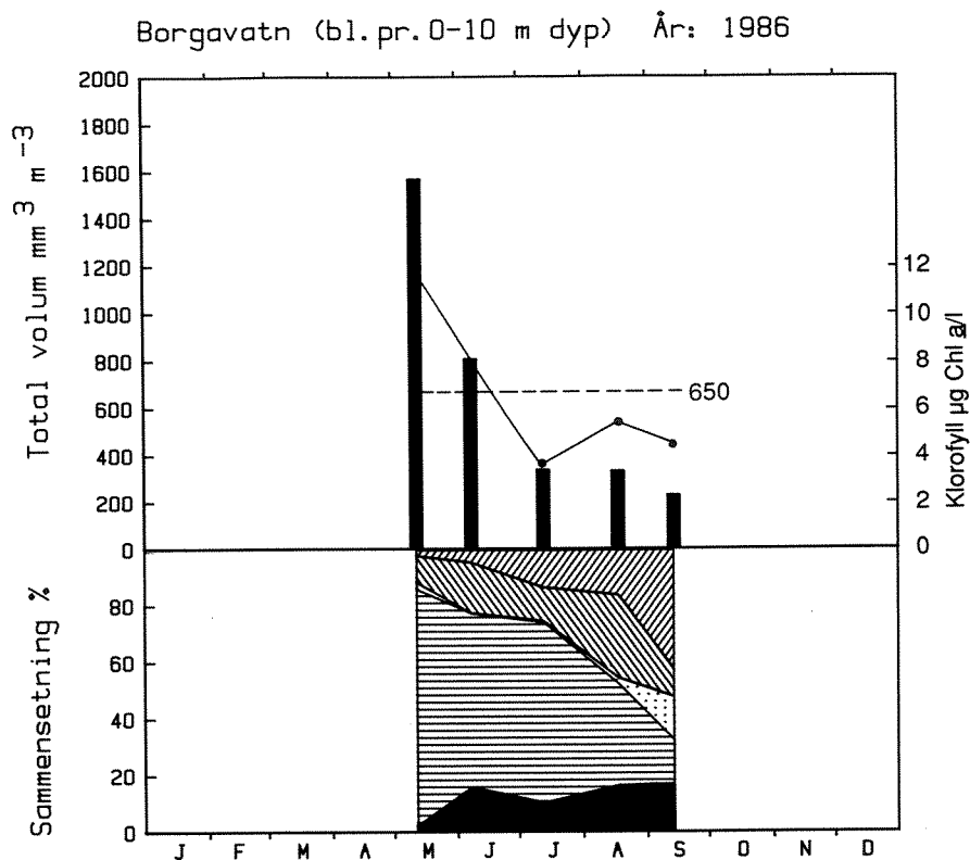
Fig. 15. Variasjoner i totalvolum og sammensetning av planteplankton i Borgevann i vekstsesongen i 1986.
