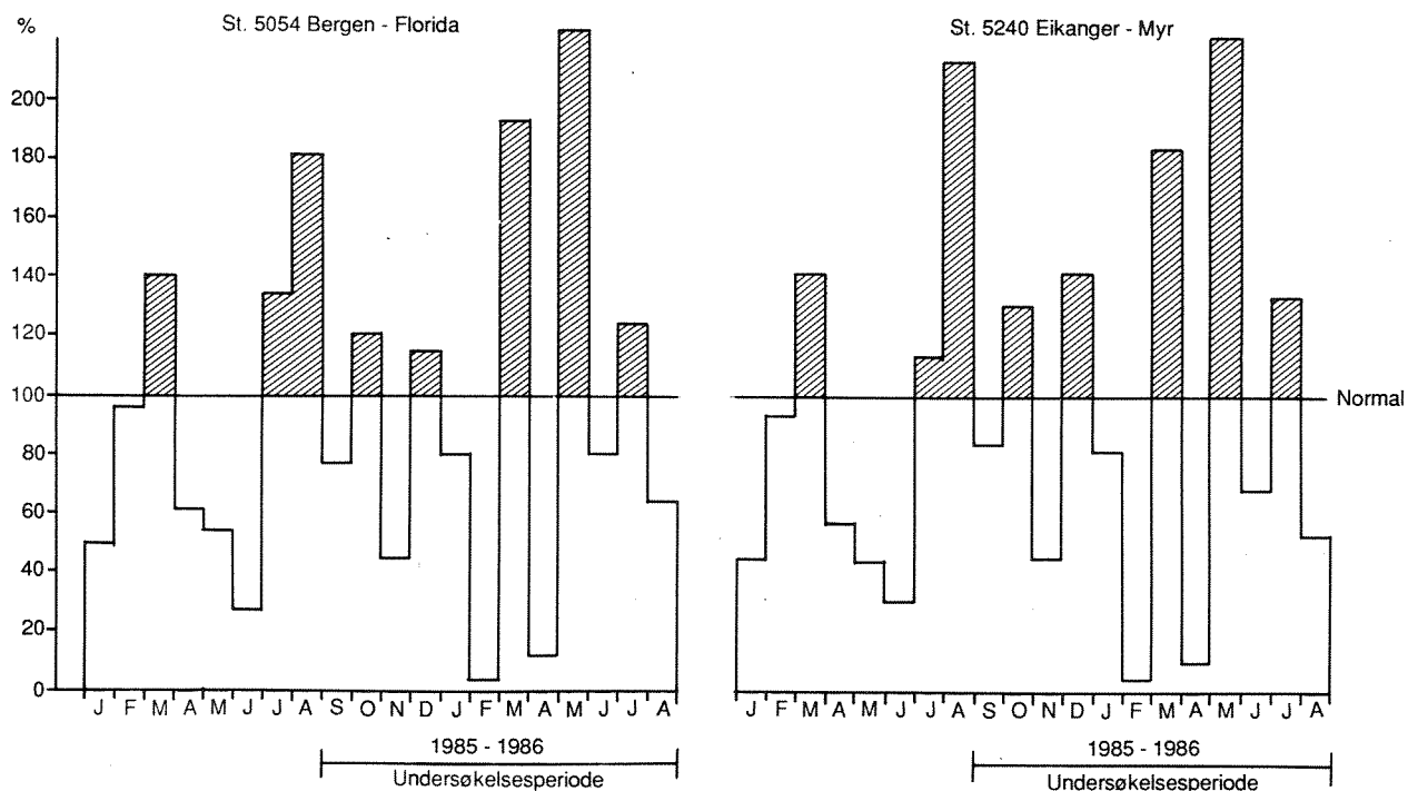
Fig. 3 B. Månedlige nedbørsummer sammenliknet med tilsvarende normalverdier for perioden 1931-1960, gitt i prosent. St. 5054 Bergen-Florida og St. 5240 Eikanger-Myr.
