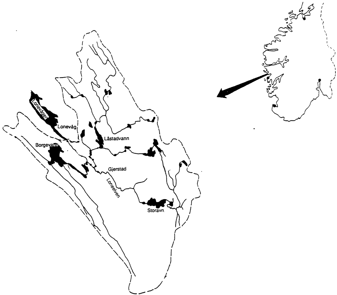
Figur 1. Loneelv-vassdragets lokalisering.
