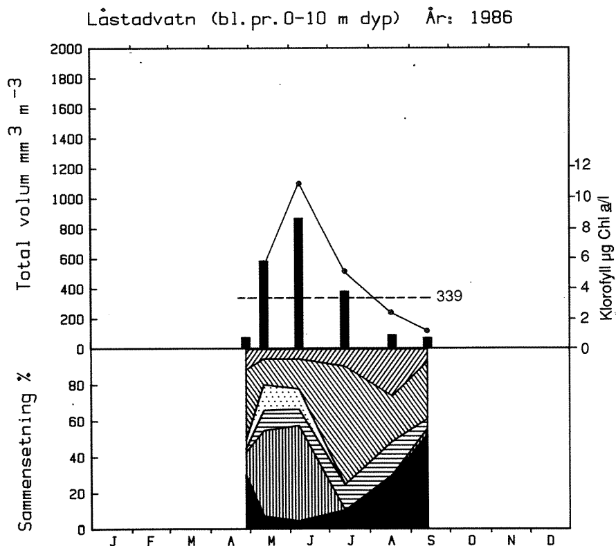
Fig. 16. Variasjoner i totalvolum og sammensetning av planteplankton i Låstadvann i vekstsesongen 1986.
