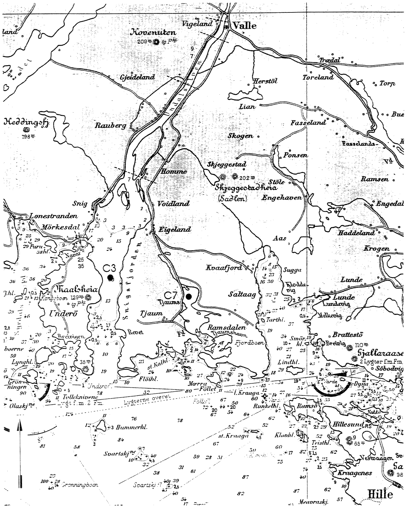
Fig. 6.1 Hydrokjemiske stasjoner i Snigsfjorden.
