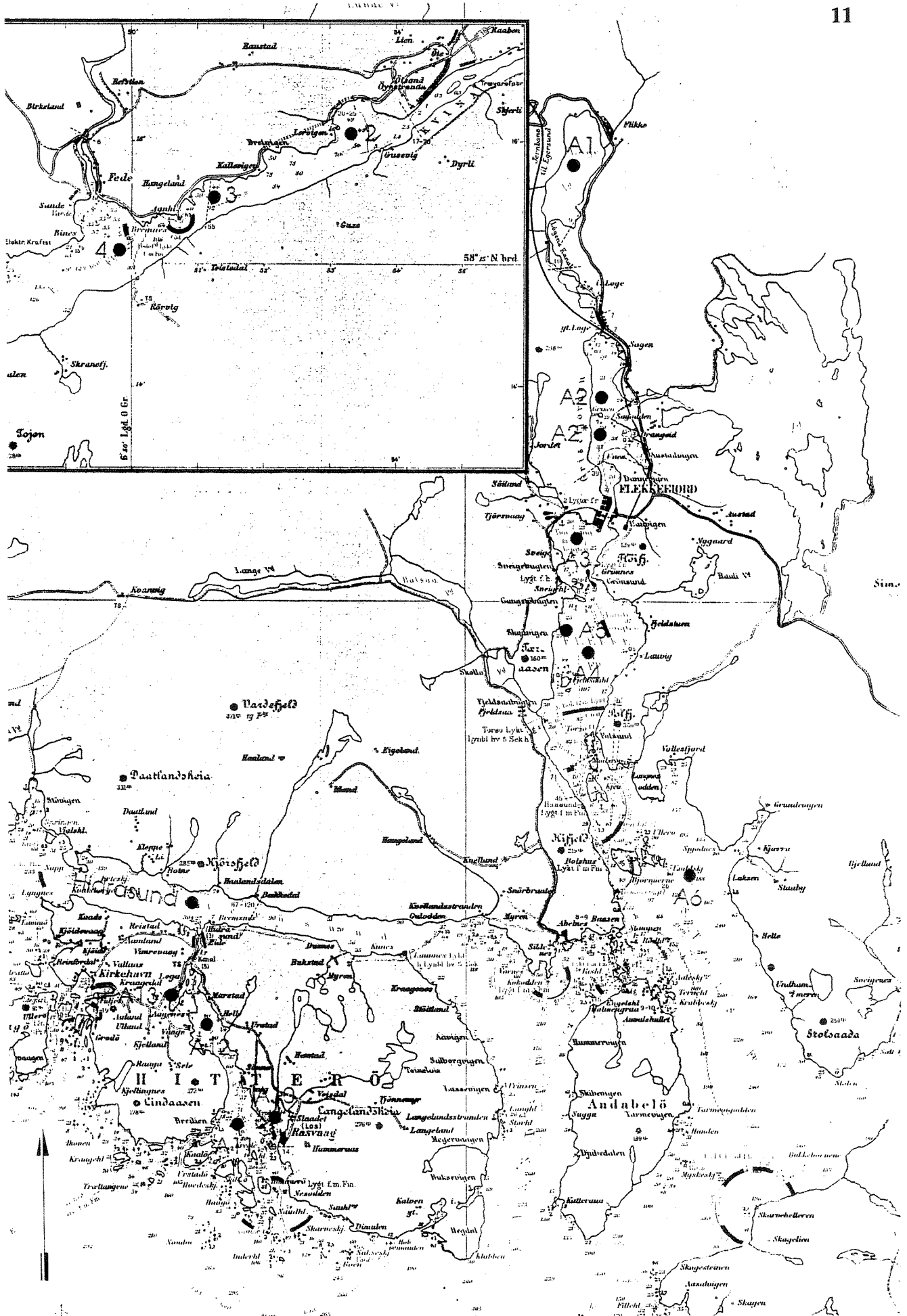
Fig. 3.1 Hydrokjemistasjoner i Flekkefjordområdet.
