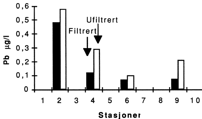
Figur 16 Bly i filtrerte og ufiltrerte prøver fra under sprangsjiktet i Ballangfjorden, 1991.
