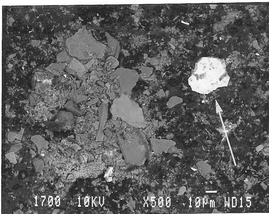
Figur 27 Aggregater av partikler fra overflatevann stasjon 4 (500x forstørrelse). Pil viser kispartikel, EDX-spekter i figur 29.
