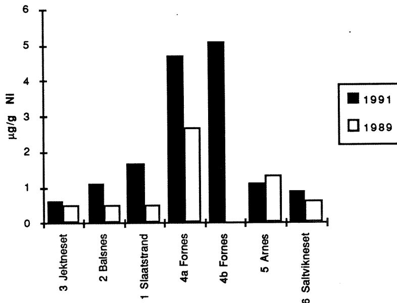
Figur 42 Innhold av nikkell i grisjetang samlet i Ballangfjorden 1989 og 1991
