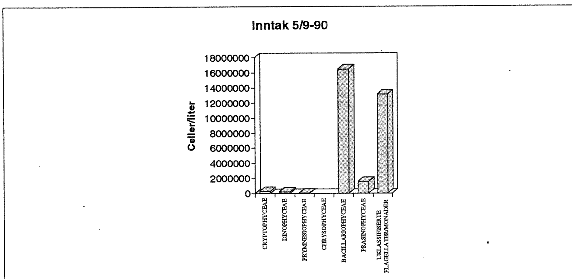
Figur 22. Den prosentvise fordeling våren 1990 basert på celletall av algeklassene i dyrkningskaret med inntaksvann som vekstmedium.
