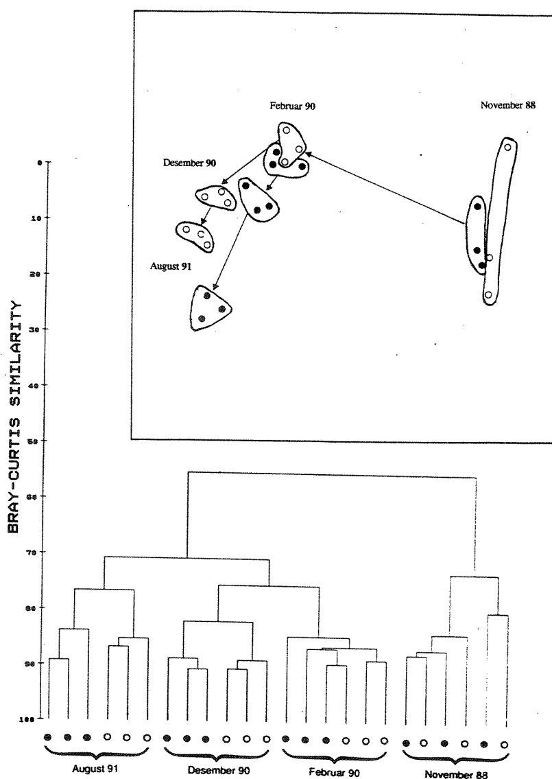
Figur 37. Dendrogram og MDS fra K over samfunnsstruktur i de fire innsamlingsperiodene november 1988 til august 1991. Åpne sirkler er bassengserie 1. Lukkete sirkler er serie 2.
