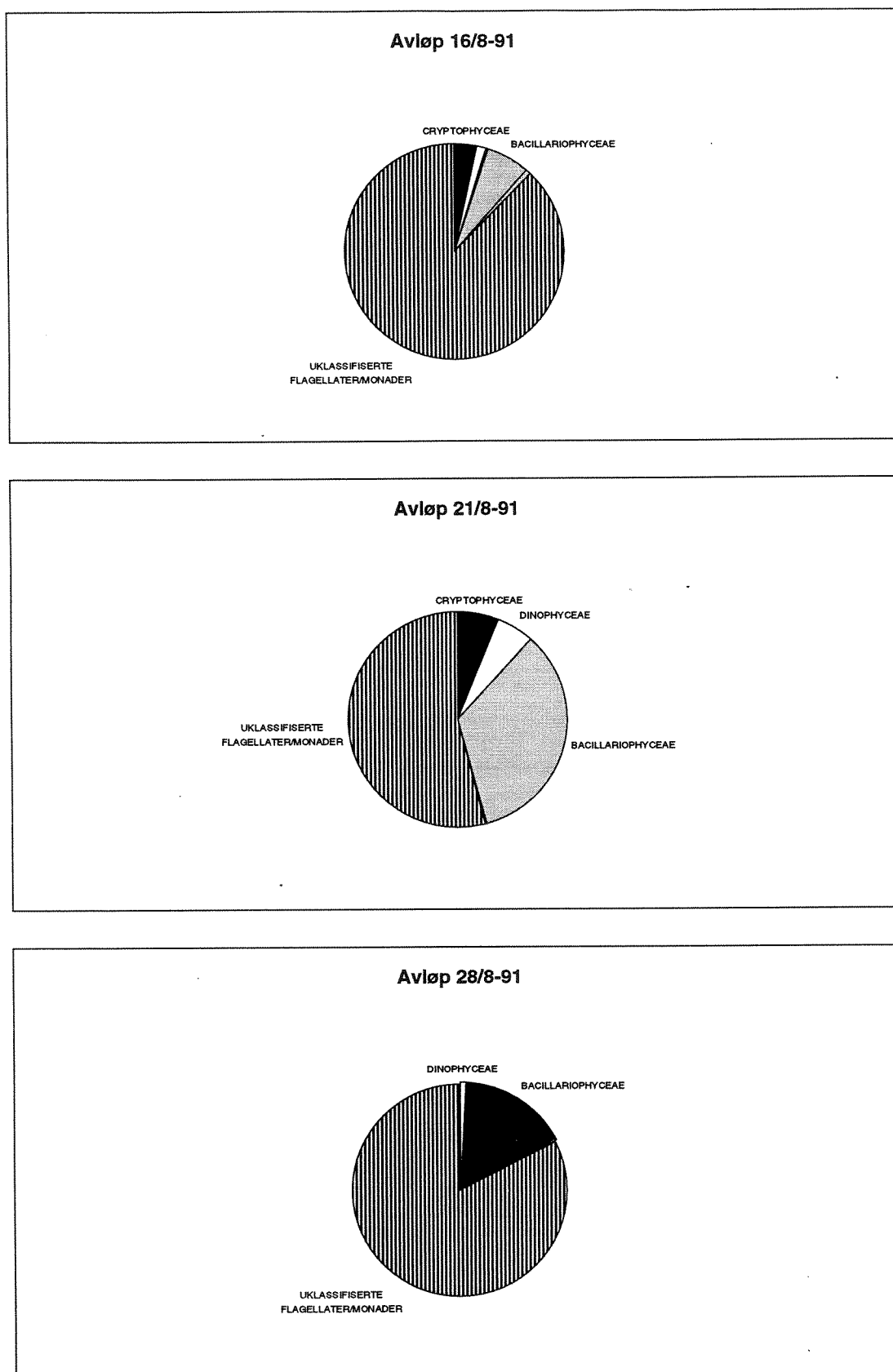
Figur 29. Den prosentvise fordeling høsten 1991 basert på celletall av algeklassene i dyrkningskaret med utløpsvann som vekstmedium.
