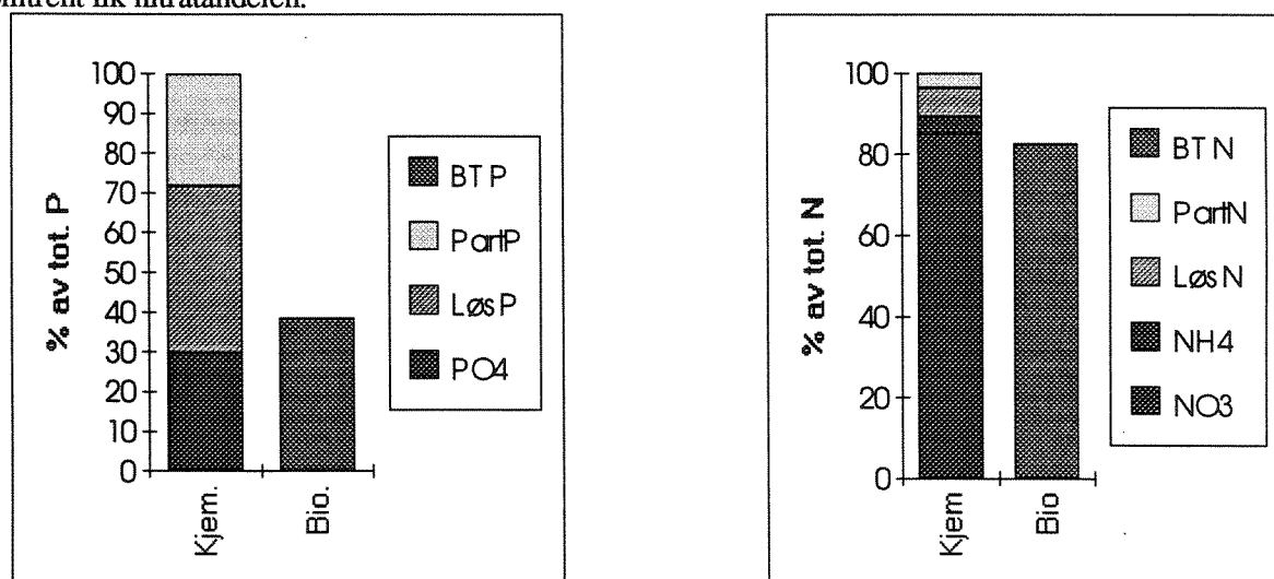
Figur 4. Middelerverdier for andelen av ulike fosfor og nitrogenfraksjoner i prøver fra landbrukspåvirkede vassdrag i mars 1991. Tot.P= 130 µg/l, tot. N= 3.5 mg/l.
