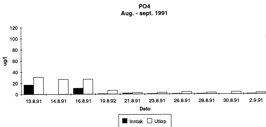
Figur 12. Fosfatutviklingen i dyrkningskarene under forsøkene i a) mai 1990, b) august/september 1990 og c) august/september 1991.
