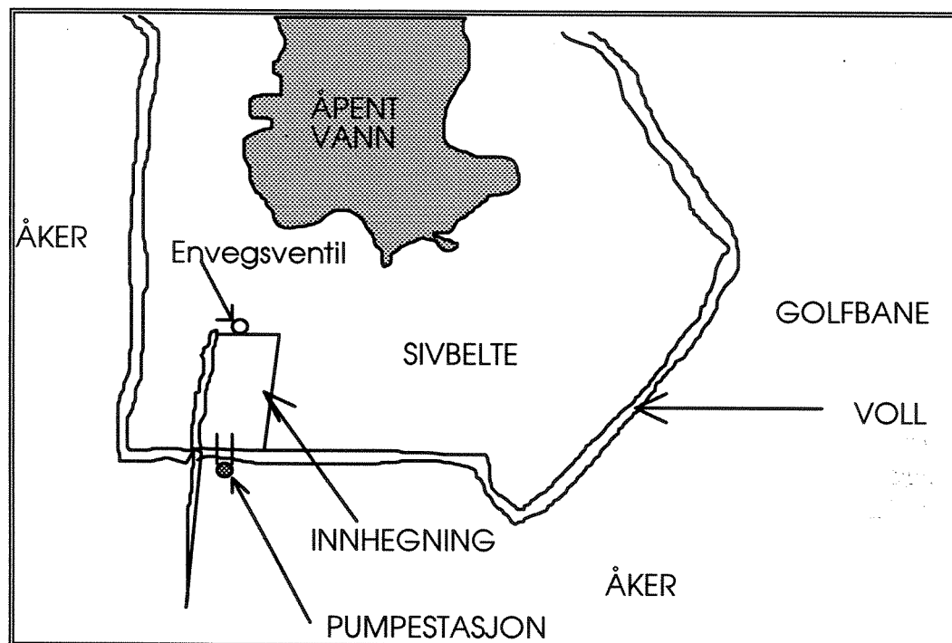
Figur 7.1 Prinsippskisse over mulig innhegning i Vassbånn's sivbelte.
