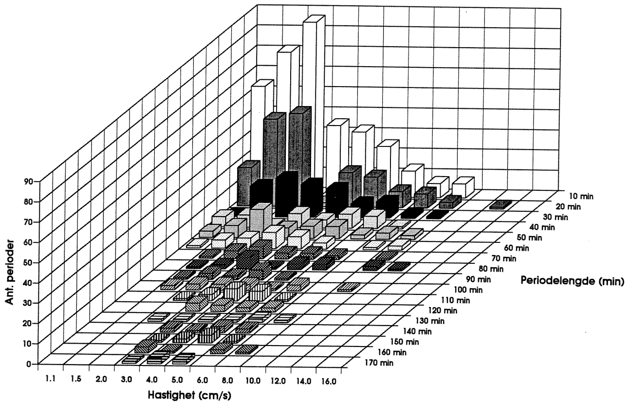
Fig. 5.2. Resultat av varighetsanalyse for strømmålingene ved Fiskerihamna i juni og oktober 1992. Kvar måleserie er inspisert med h.t. forekomst av perioder med strøm vedvarande under gjevne strømgrensar. Antallet slike perioder med gitt varigheit er talt opp, og presentert i matriseform.
