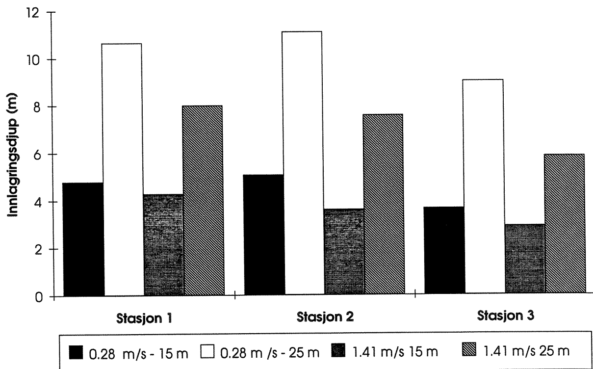
Fig. 4.1. Resultat (middelverdiar for alle hydrografiske profilar på kvar stasjon) for innlagringsdjup, ved variert fluks (utgangsfart) og utsleppsdjup.
