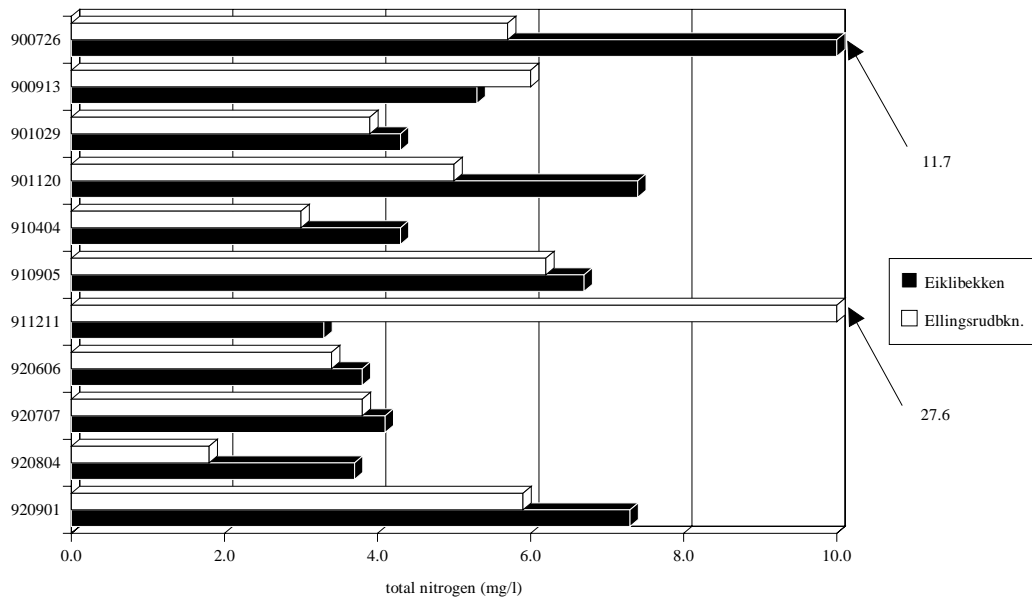
Figur 3.15 Total nitrogen i Finstadbekken og Ellingsrubbekken
