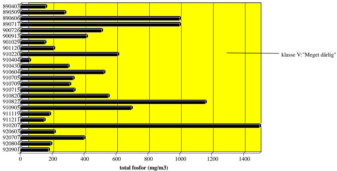
Figur 3.5 Fosforregistreringer ved st. 2 (utløp kulvert i Blåveisbekken ved Hebekk)
