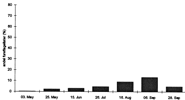
Figur 3.13 Andel fureflagellater 1993
