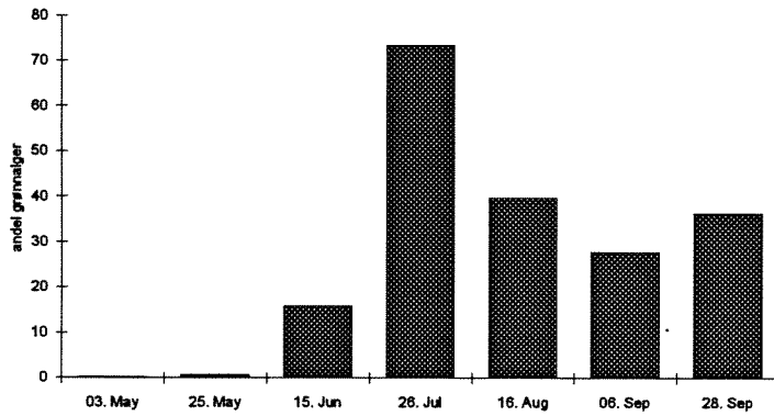
Figur 3.11 Andel grønnalger 1993
