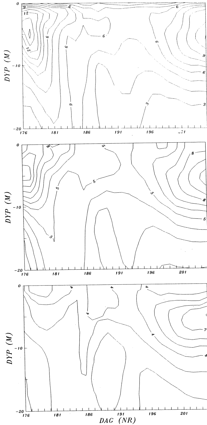
Fig. 5.14 Beregnet planktonkonsentrasjon ( \text{mg P/m}^3 ) i a) indre, b) midtre og c) ytre Glomfjord.
