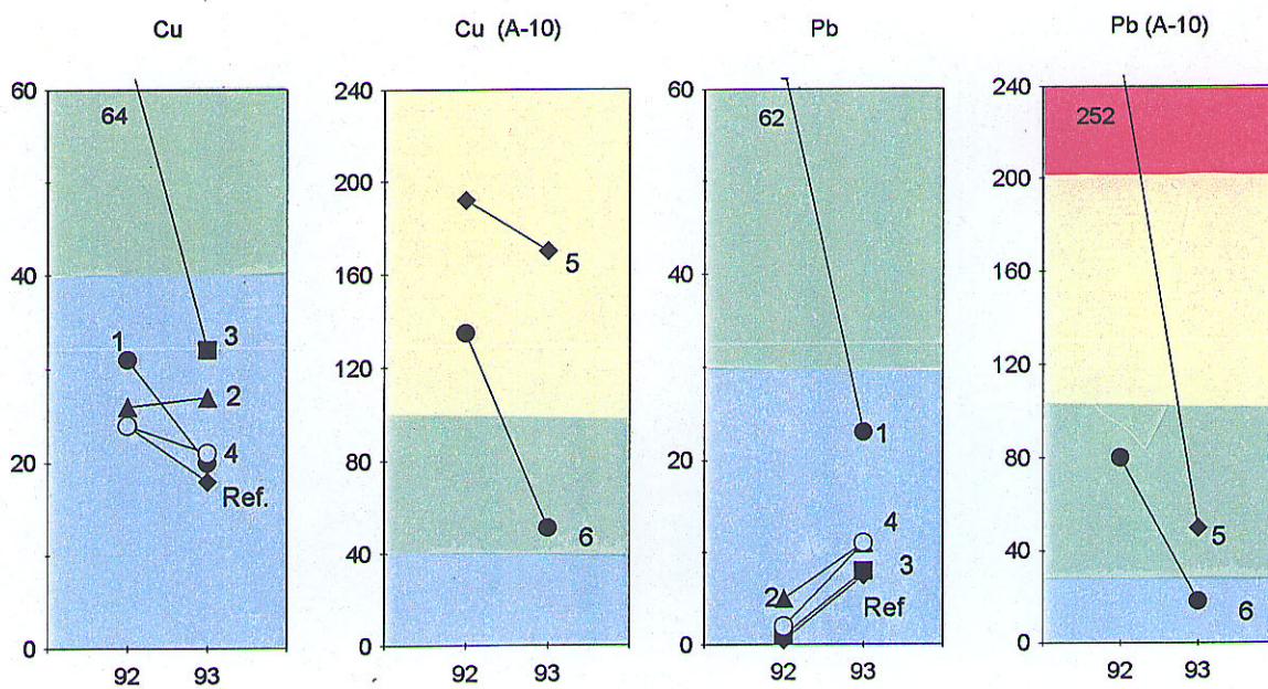
Fig.17. Konsentrasjoner (µg/g T.V.) i mose på stasjonene i Sætermoen og Karlstadskogen skytefelt.
