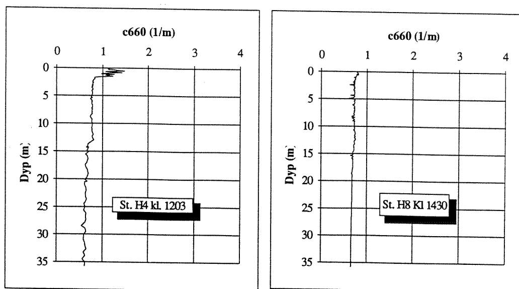
Fig.3.8. Transmisjonsprofiler uttrykt som svekningskoeffisienten, c_{660} ( m^{-1} ) for stasjon H4 og H8 den 17. august 1994 i Holandsfjorden.
