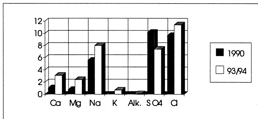
Fig 9. Hallevann. Hovedkomponenter, mg/l, 1990 og 1993/94
