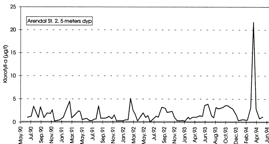
Figur 35. Klorofyll-a ved Arendal St. 2 på 5 meters dyp mai 1990 til mai 1994..
