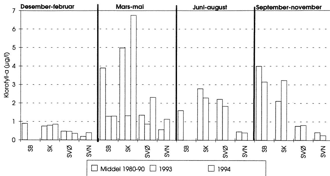
Figur 30. Midlere klorofyllkonsentrasjon ved Arendalstasjonene i ulike vannmasser etter sesong 1993-mai 1994, sammenlignet med sesongsmiddelkonsentrasjonen fra perioden 1980-90. (Data fra 1980-90 fra HFF).
