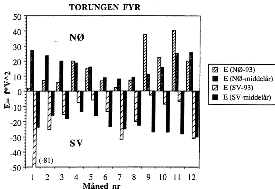
Figur 4. Vindforholdene (E) langs sørlandskysten 1993 sammenlignet med 1961-90. ( E=fv^2 , hvor f =frekvensen og v =m/s). (Data fra Meteorologisk institutt).
