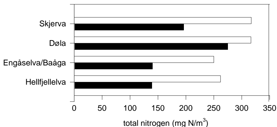
Figur 4.3 Målte konsentrasjoner av fosfor og nitrogen (hvite stolper) i de fire hovedvassdragene sammenliknet med beregnede verdier ut fra foreliggende informasjon om forurensningskilder (svarte stolper)
