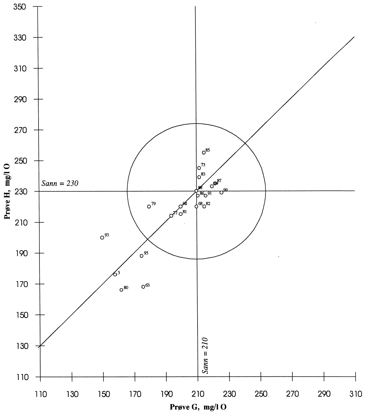
Fig. 10. Biokjemisk oksygenforbruk
