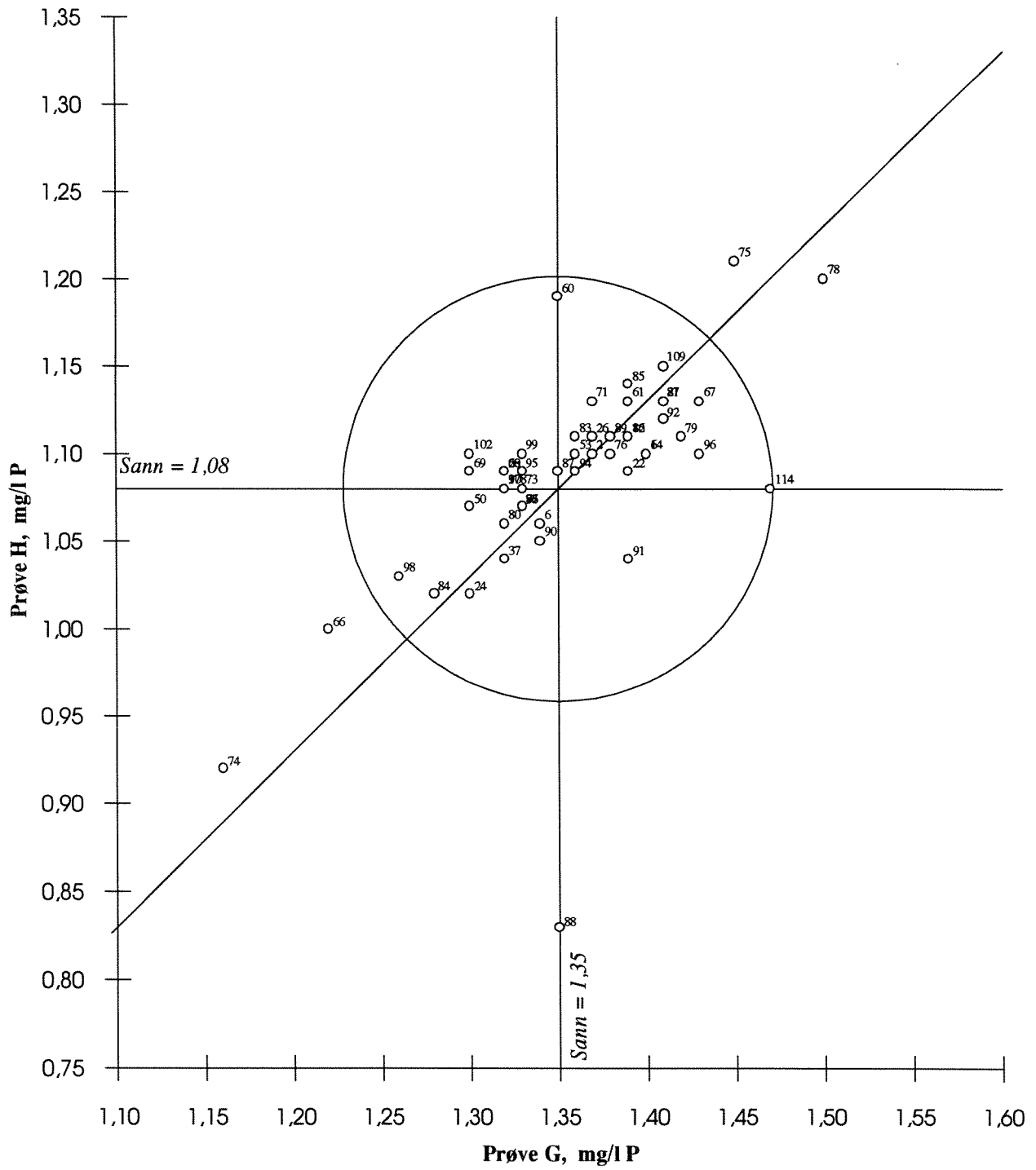
Fig. 14. Totalfosfor
