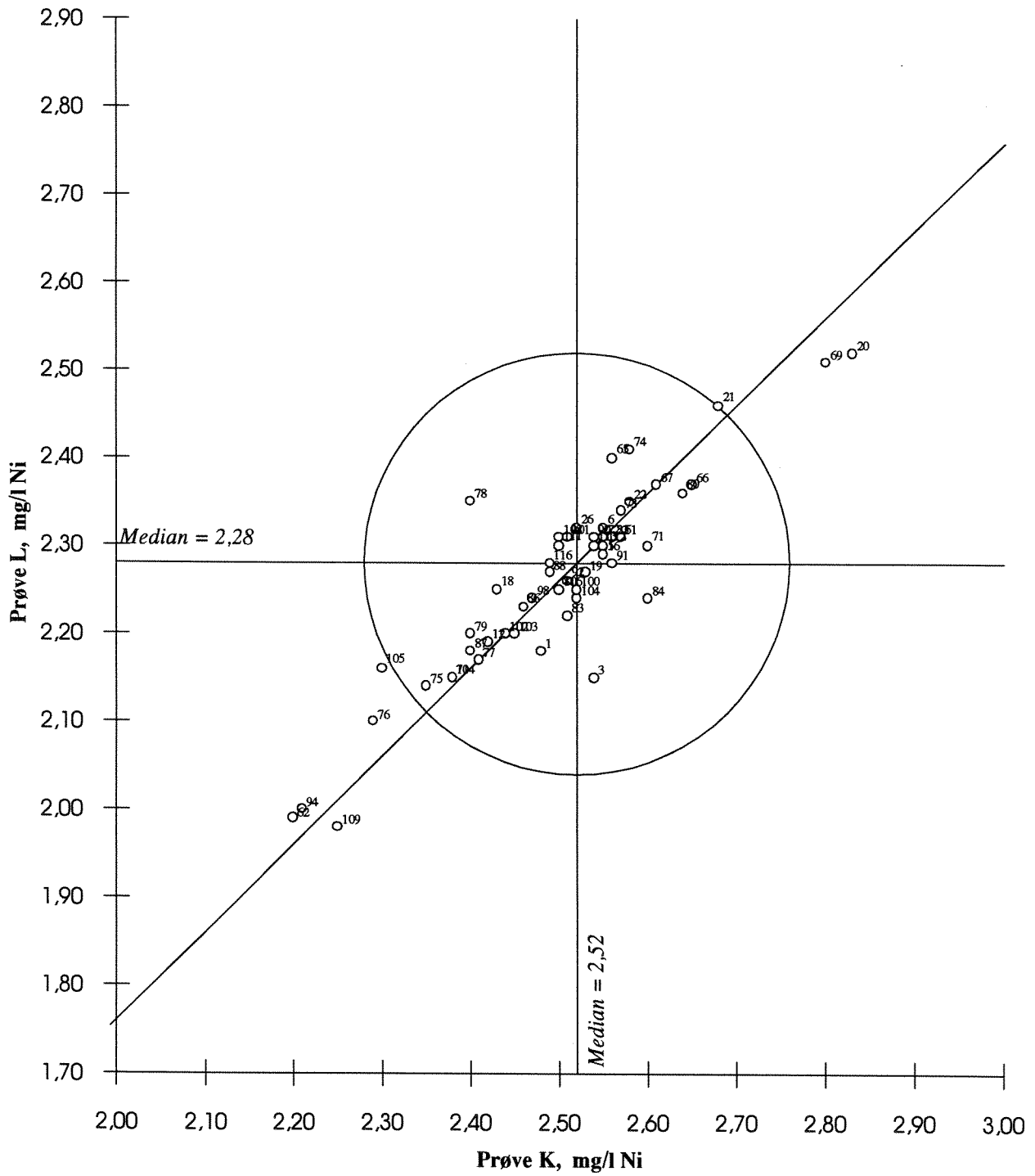
Fig. 30. Nikkel
