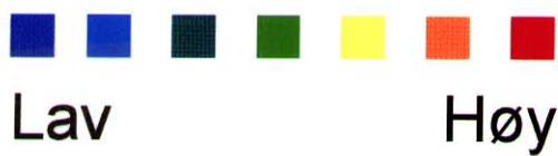
Fig. 3.13. Satellittbildet viser den relative temperaturfordelingen i de øvre vannmasser av Byfjorden og de nærmeste fjordene den 6. juni 1990. Satellittdataene er bearbejdet av NIVA på basis av data fra Thematic Mapper sensoren TM6 ombord i jordressurssatelitten Landsat-5.
