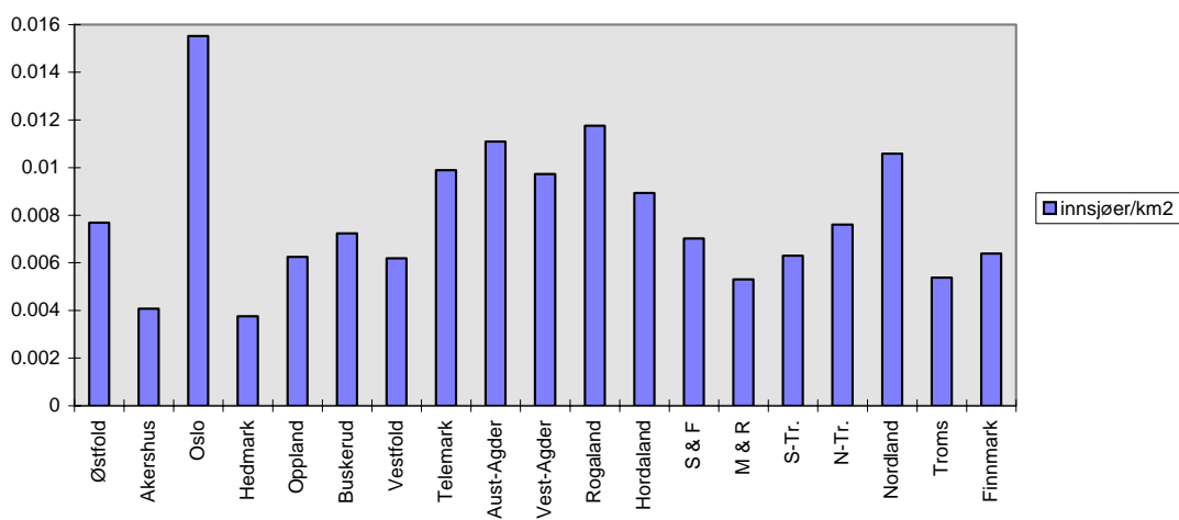
Figur 3.6. Tetthet av innsjøer større enn 1 km 2 pr. fylke
