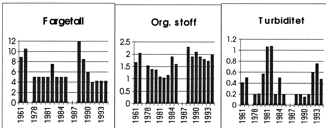
Fig. 8.4. Årsmiddeler for fargetall (mg Pt/l), org. stoff ( COD_{Mn} (mg O/l) før 1988 og TOC (mg C/l) etter 1988) og turbiditet (mg SiO 2 /l i 61/62, senere FTU).
