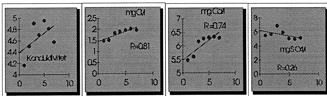
Fig 7.5. Tidstrender fra 1988 (0) til 1994 (7). Konsentrasjoner langs y-aksen.
