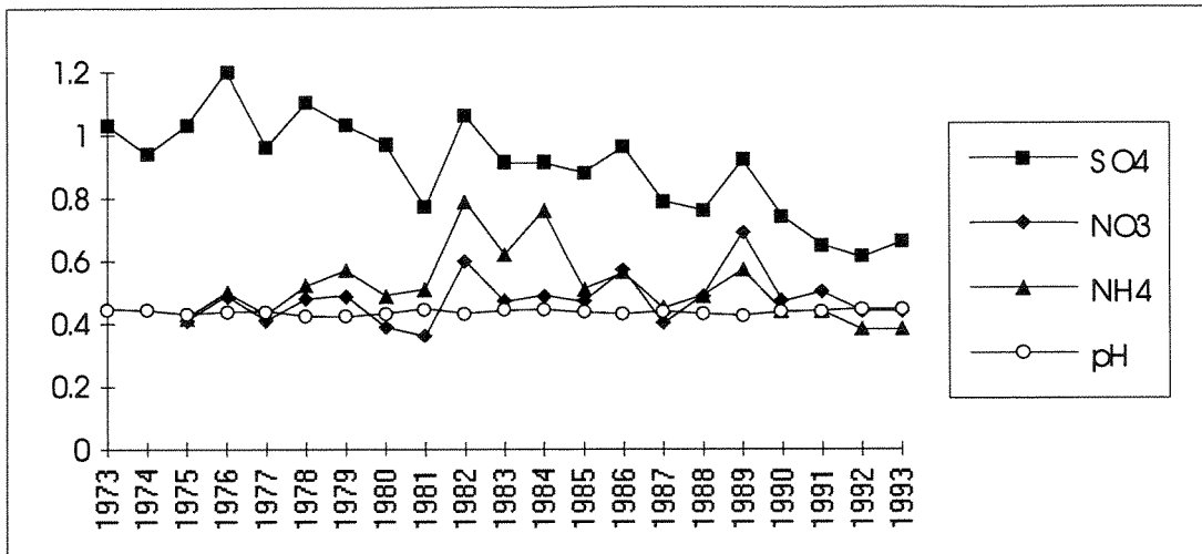
Fig. 4.4. Løken, Trøgstad. Årsmiddelkonsentrasjoner for sulfat, nitrogenforbindelser og pH. Benevning: mg SO 4 /l, NO 3 -mg N/l, NH 4 -mg N/l og pH 0.1.
