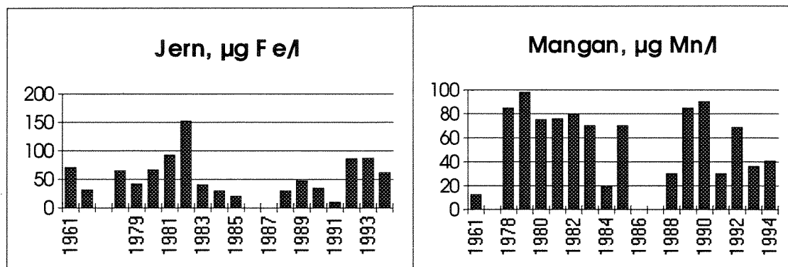
Fig. 8.3. Årsmiddeler for jern og mangan.
