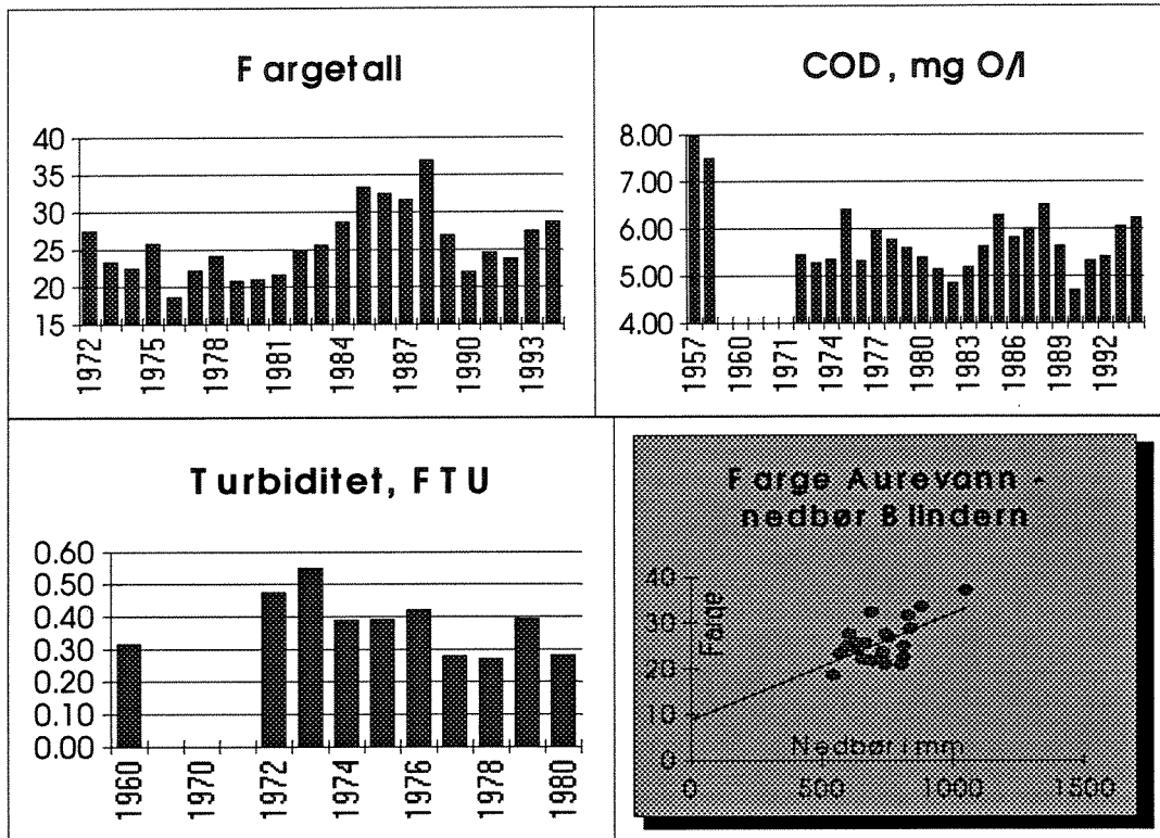
Fig. 6.8. Fargetall (mg Pt/l), COD_{Mn} (mg O/l), turbiditet og forhold farge - nedbør.
