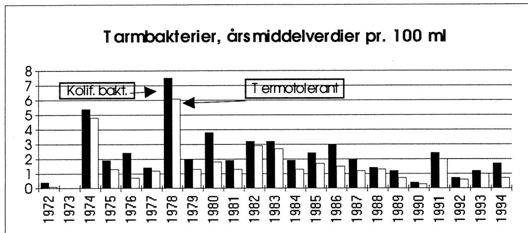
Fig. 7.11. Årsmiddelverdier for tarmbakterier pr. 100 ml.
