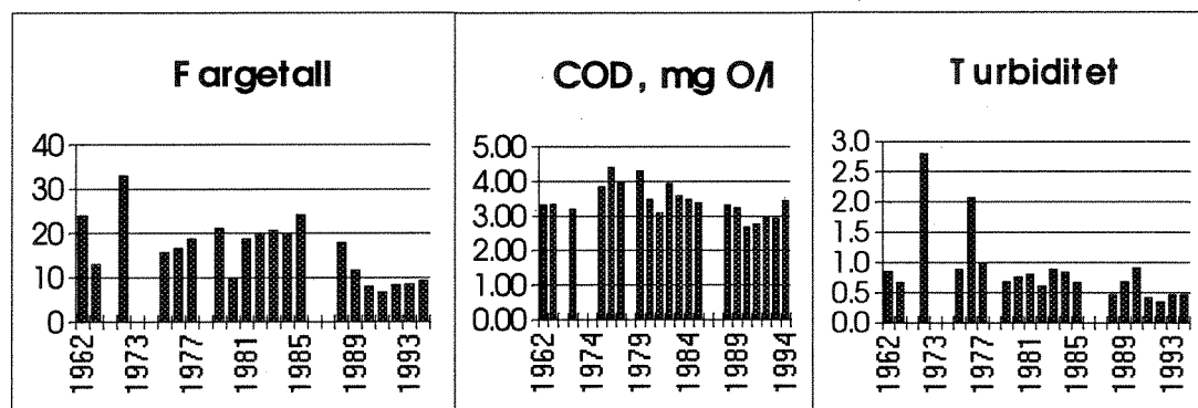
Fig. 7.7. Årsmiddelverdier for fargetall (mg Pt/l), COD_{Mn} og turbiditet (FTU).
