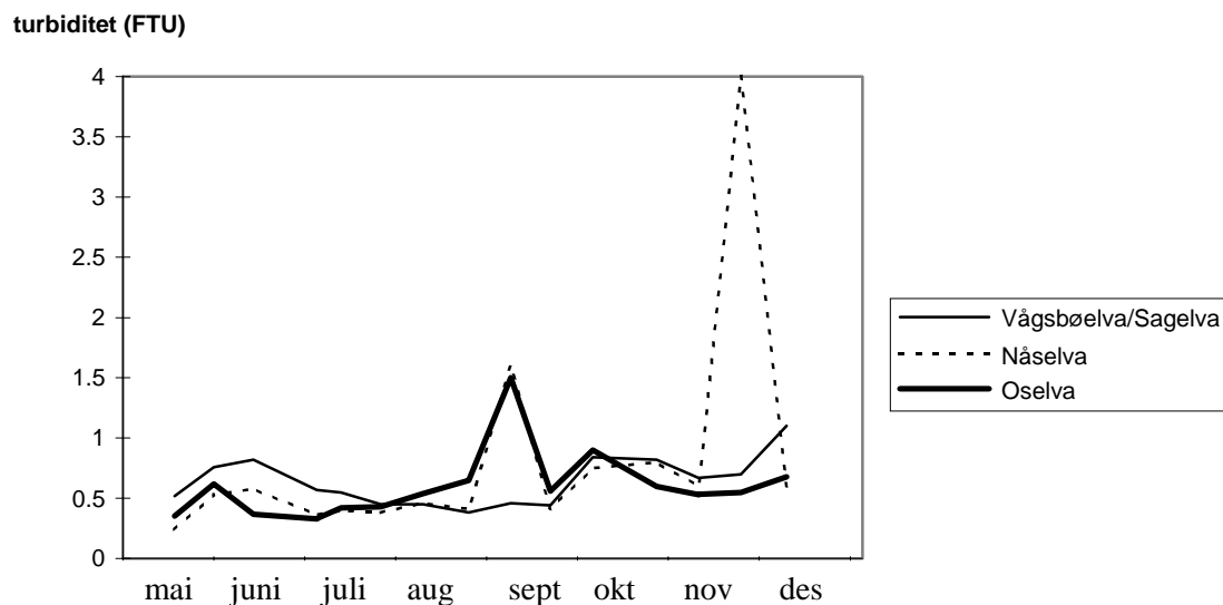
Figur 3.2.3 Turbiditet i de tre målte bekkene
