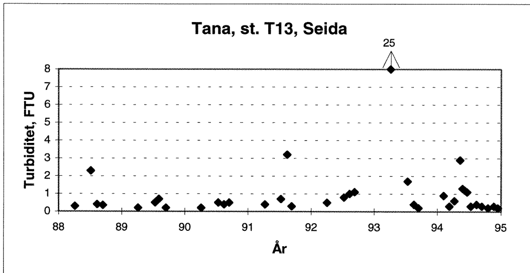
Figur 2.2. Turbiditet i Tanaelva ved Seida, st.T13.
