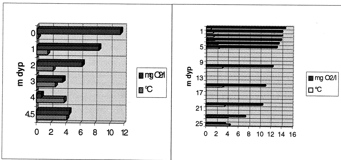
Fig. 5.1. Kjerkevatn. Temperatur og oksygen 13./14. april 1994.
