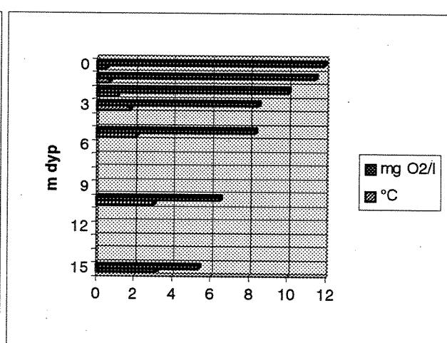
Fig. 5.6. Kjerkhaugv. Temperatur og oksygen 13./14. april 1994
