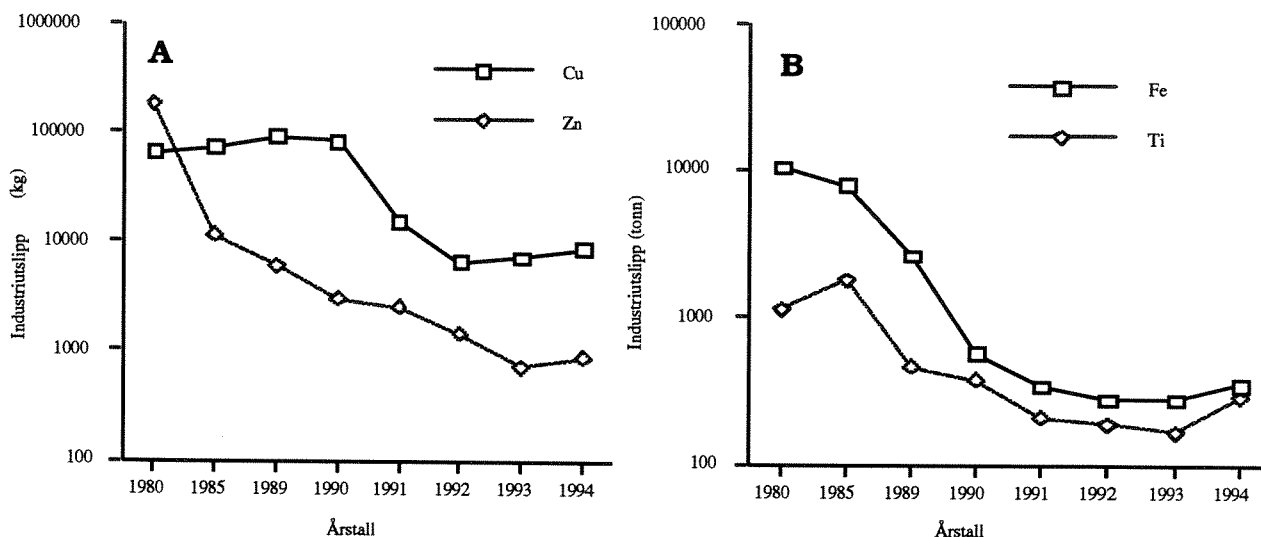
Figur 4.1. Samlede industriutslipp (log-skala) av kobber og sink (A) og jern og titan (B) fra Sarpsborg og Fredrikstad-området (data bearbejdet etter Holtan, 1996). Merk at enheter på y-aksen er forskjellig i A og B.
