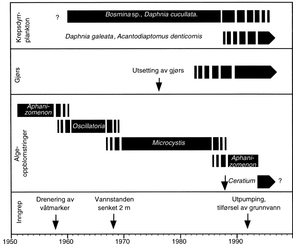
Figur 14. Skjematisert illustrering av de viktigste endringene i Akersvannets økosystem.
