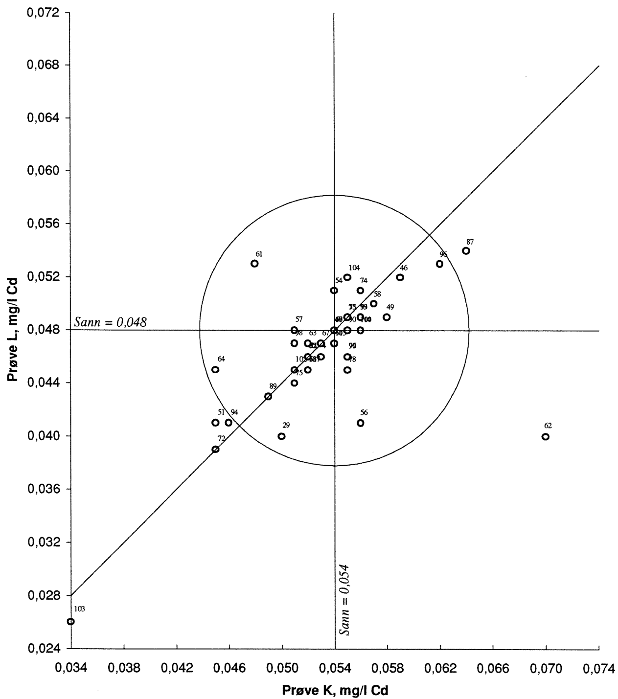
Figur 22. Youdendiagram for kadmium, prøvepar KL Akseptansegrensen, angitt med en sirkel, er 20 %
