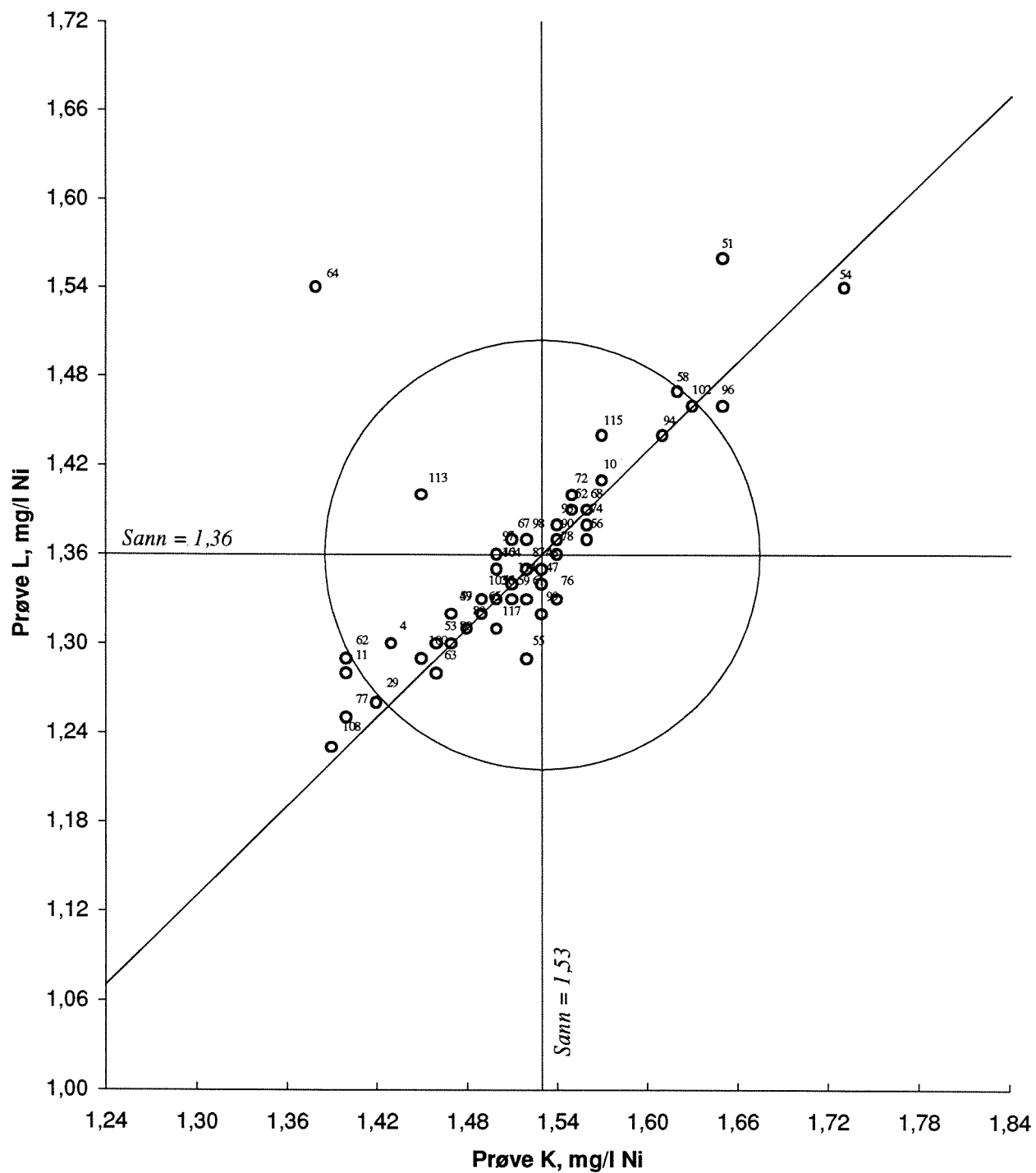
Figur 30. Youndendiagram for nikkel, prøvepar KL Akseptansegrensen, angitt med en sirkel, er 10 %
