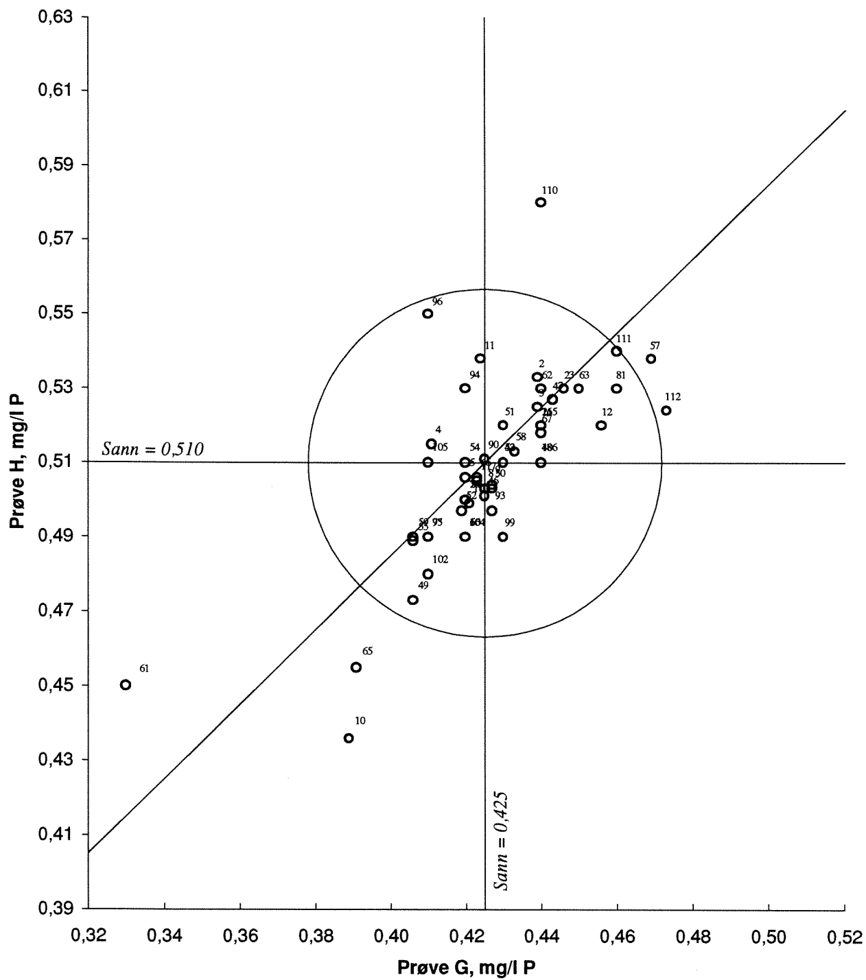
Figur 12. Youdendigram for totalfosfor, prøvepar GH Akseptansegrensen, angitt med en sirkel, er 10 %
