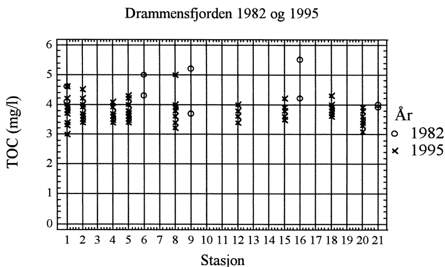
Figur 16. TOC (mg/l) i overflatevann somrene 1982 og 1995.
