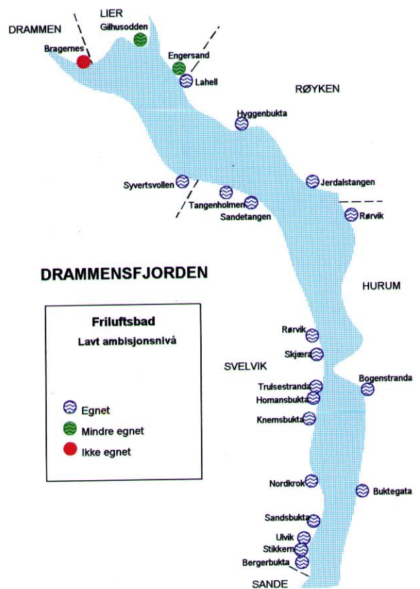
Figur 8. Egnethet for friluftsbad i Drammensfjorden i 1982, 1991 og 1995 bedømt etter termotolerante koliforme bakterier, samt laveste ambisjonsnivå for friluftsbad ved ulike badeplasser (Sørensen m.fl., 1995).
