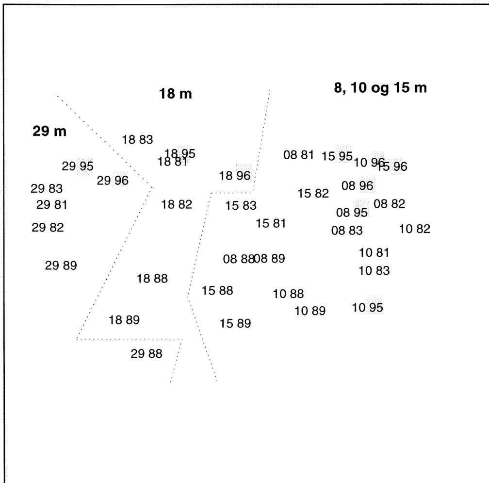
Figur 38. Stereostasjon K4, Vaagaholmen. Stasjonsbeliggenhet og MDS-plott for hvert dyp for hele perioden 1981-96. Stiplet linje: gruppering mellom stasjoner. Stress: 0.13.
