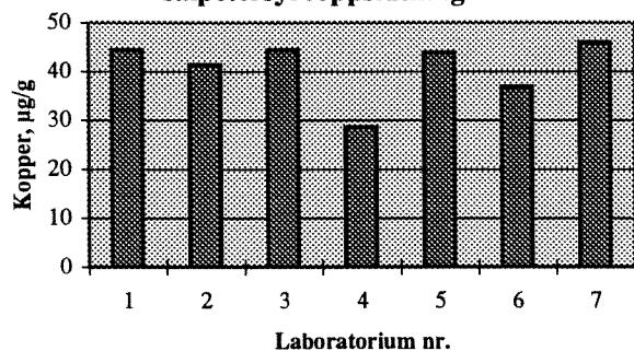
Fig. 6a, kopper i prøve C, salpetersyreoppslutning
