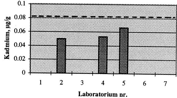
Fig. 3b, kadmium i prøve B, totaloppslutning
