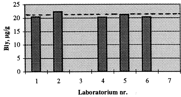
Fig. 9b, bly i prøve B, totaloppslutning
