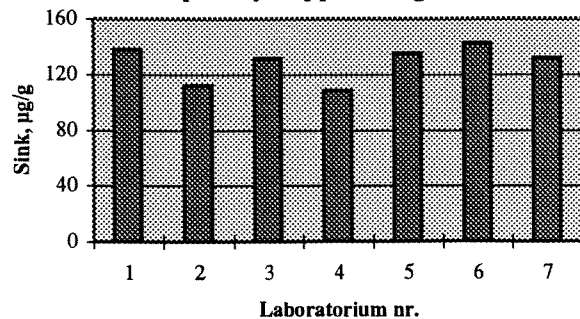
Fig. 8a, sink i prøve C, salpetersyreoppslutning
