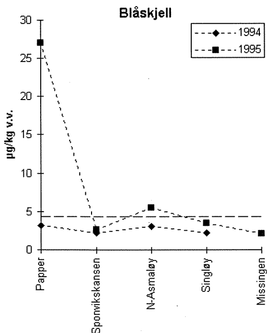
Figur 6. Konsentrasjonen av \Sigma\text{PCB}_7 (summen av PCB-28, PCB-52, PCB-101, PCB-118, PCB-153, PCB-138, , PCB-180) i blåskjell fra 5 stasjoner i Hvaler området før og etter storflommen i Glomma i 1995. Horisontal prikket linje antyder foreslått høyt bakgrunnsnivå i bare diffust belastede områder (Knutzen og Green, 1995).
