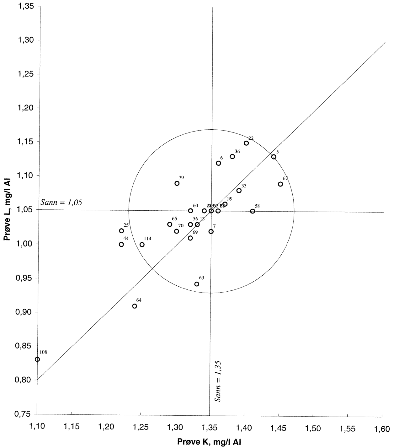
Figur 16. Youdendiagram for aluminium, prøvepar KL Akseptansgrensen, angitt med en sirkel, er 10 %
