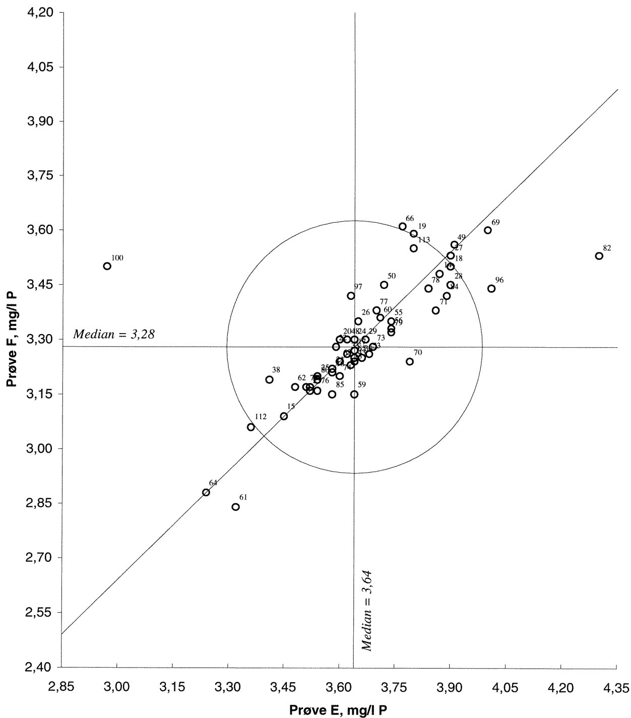
Figur 11. Youdendiagram for totalfosfor, prøvepar EF Akseptansegrensen, angitt med en sirkel, er 10 %
