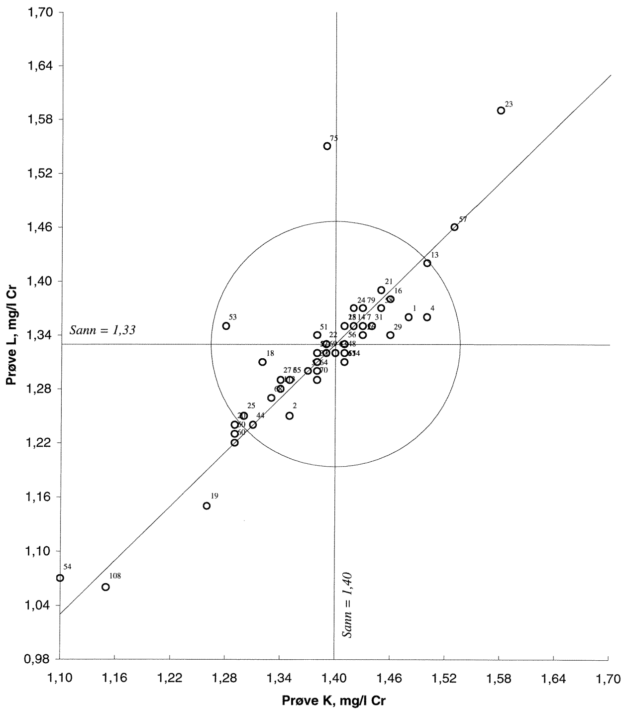
Figur 26. Youdendiagram for krom, prøvepar KL Akseptansegrensen, angitt med en sirkel, er 10 %
