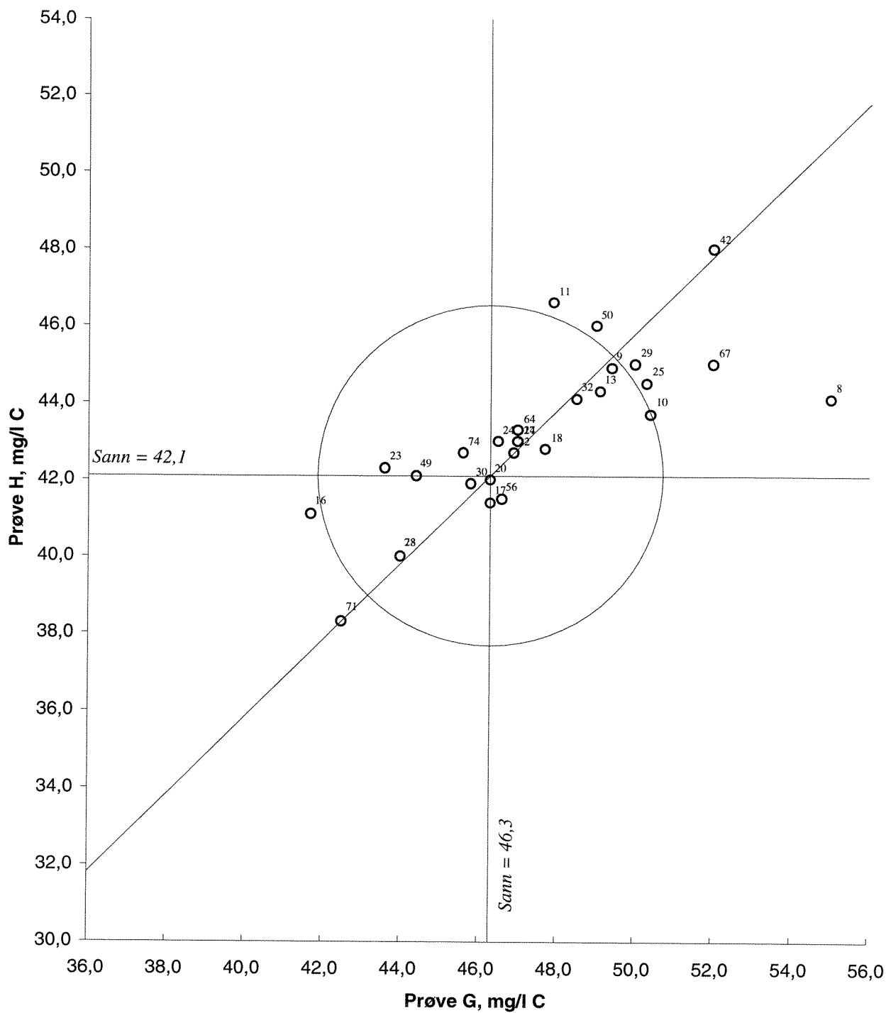
Figur 10. Youdendiagram for totalt organisk karbon, prøvepar GH Akseptansegrensen, angitt med en sirkel, er 10 %
