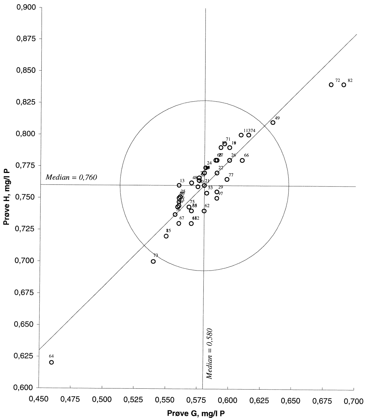
Figur 12. Youndendiagram for totalfosfor, prøvepar GH Akseptansegrensen, angitt med en sirkel, er 10 %
