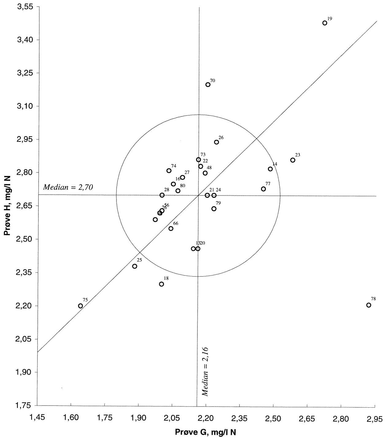
Figur 14. Youtendigram for totalnitrogen, prøvepar GH Akseptansegrensen, angitt med en sirkel, er 15 %
