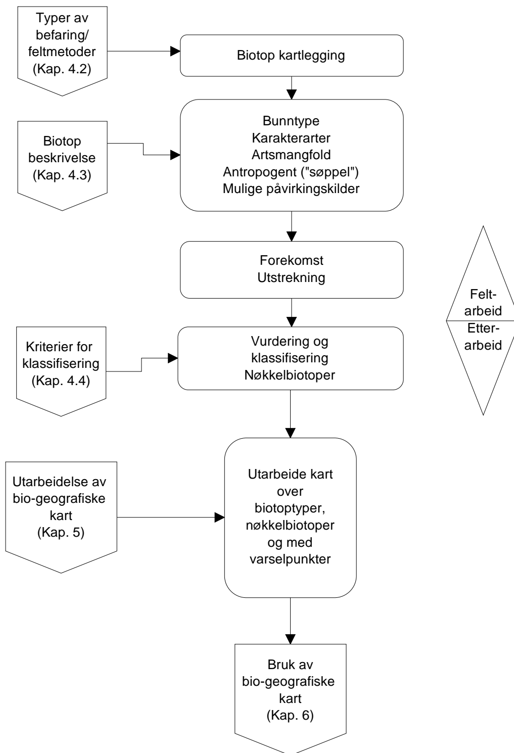
Figur 3. Skjematisk framstilling av de ulike elementer som inngår i framstillingen av et biotopkart over marine gruntvannsrområder.
