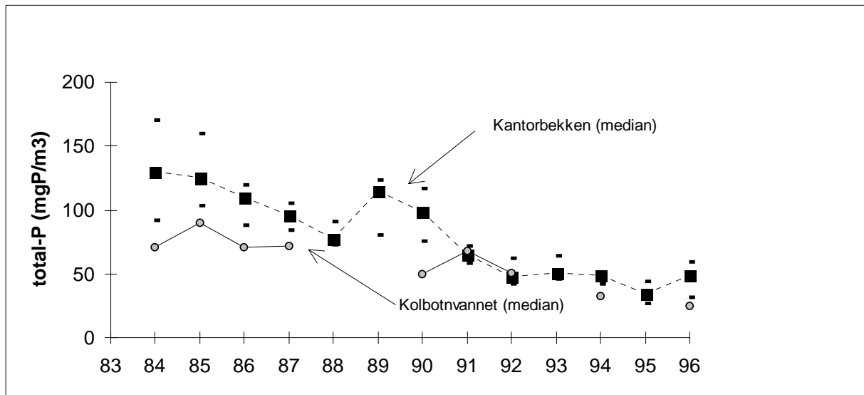
Figur 7.1 Årsverdier for total-fosfor i Kolbotnvannet og i utløpsbekken Kantorbekken. verdiene er medianer, dvs. at halvparten av resultatene fra ett år er større enn medianen, og den andre halvparten er mindre. De vertikale linjene angir det området der vi finner 50 % av resultatene for hvert år i Kantorbekken.
