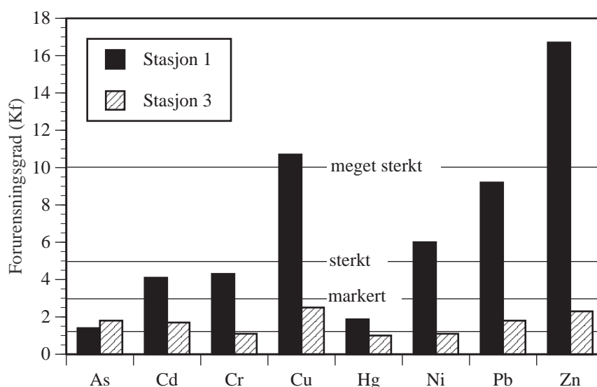
Figur 7.2.2. Forurensingsgrad eller kontamineringsfaktor (Kf) for de ulike tungmetallene målt i sedimentene fra de to stasjonene i Kolbotnvann. Kontamineringsfaktoren er lik forholdet mellom konsentrasjonen i overflatesedimentet og referansesedimentet.
