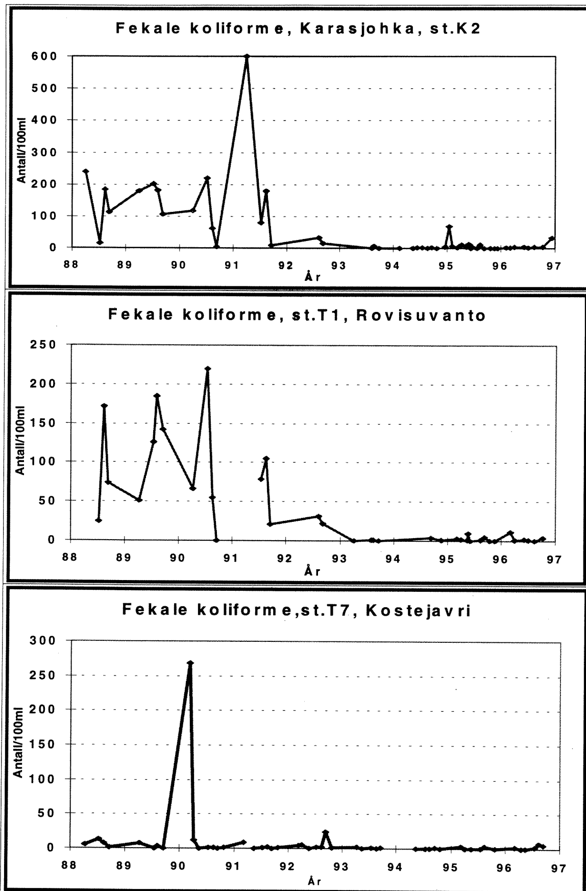
Figur 3.1. Fekale koliforme bakterier ved Karasjohka (K2), Rovisuvanto (T01) og Kostejavri (T07), 1988 -1996.
