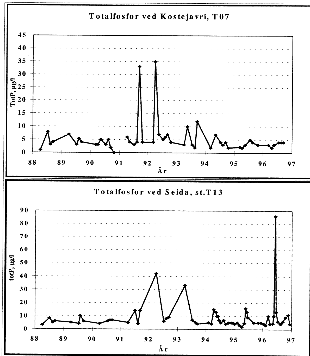
Figur 2.4. Totalfosfor ved Kostejavri og Seida .
