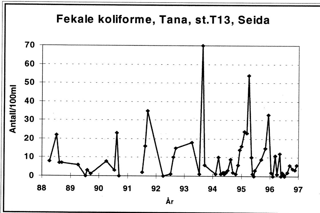
Figur 3.2. Fekale koliforme bakterier ved Tana bru og Seida, 1988-1996.
