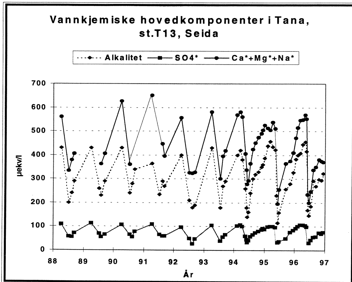
Figur 2.1. Vannkjemiske hovedkomponenter i Tana ved Seida (T13) for perioden 1988-1996. Ca* +Mg*+Na* (sjøsaltkorrigert), SO4*( sulfat, sjøsaltkorrigert) og alkalitet.
