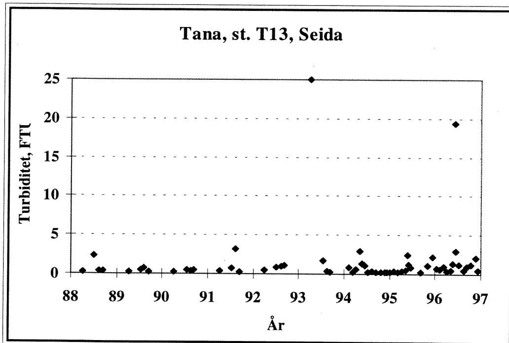
Figur 2.2. Turbiditet i Tanaelva ved Seida, st.T13.
