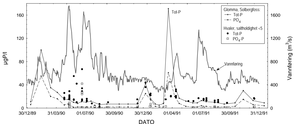
Figur 12. Sammenligning av fosfordata fra ferskt overflatevann (saltholdighet <5) i Hvalerestuaret (Magnusson og Sørensen 1993) og Glomma ved Solbergfoss fra 1990 og 1991 (Holtan et al. 1991, 1992). Vannføringsdata fra NVE.
