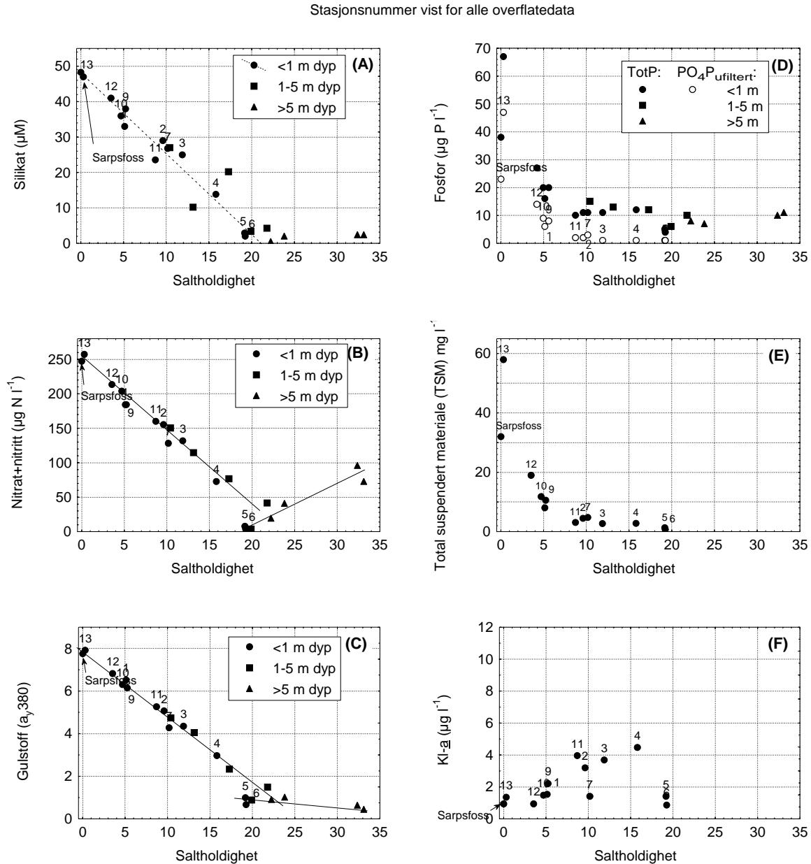
Figur 11. Stoffkonsentrasjoner mot saltholdighet i Hvalerestuariet 5. juni 1995. I Plott A - D er det vist data både fra overflaten, fra sjiktet 1-5m og fra dyp >5m (se symbolforklaring i figuren), mens det for plott E og F bare er vist data fra overflaten. Stasjonsnummer er vist for alle overflatedata.
