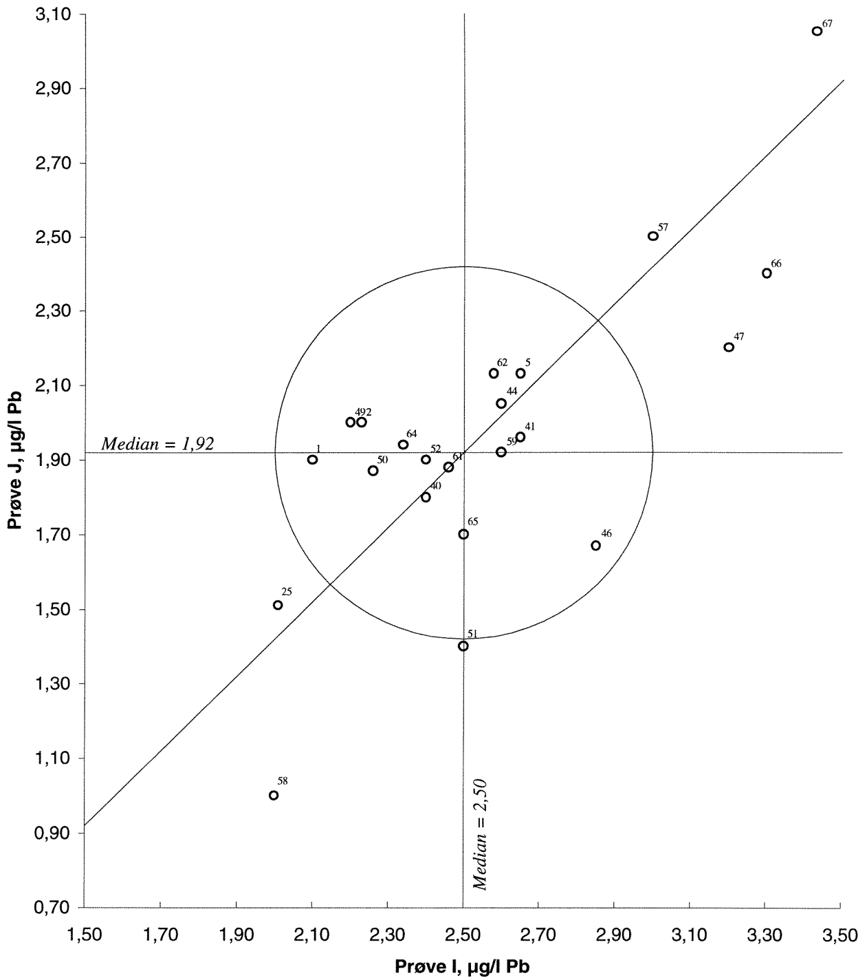
Figur 37. Youdendiagram for bly, prøvepar IJ Akseptansegrensen, angitt med en sirkel, er 0,5 µg/l Pb
