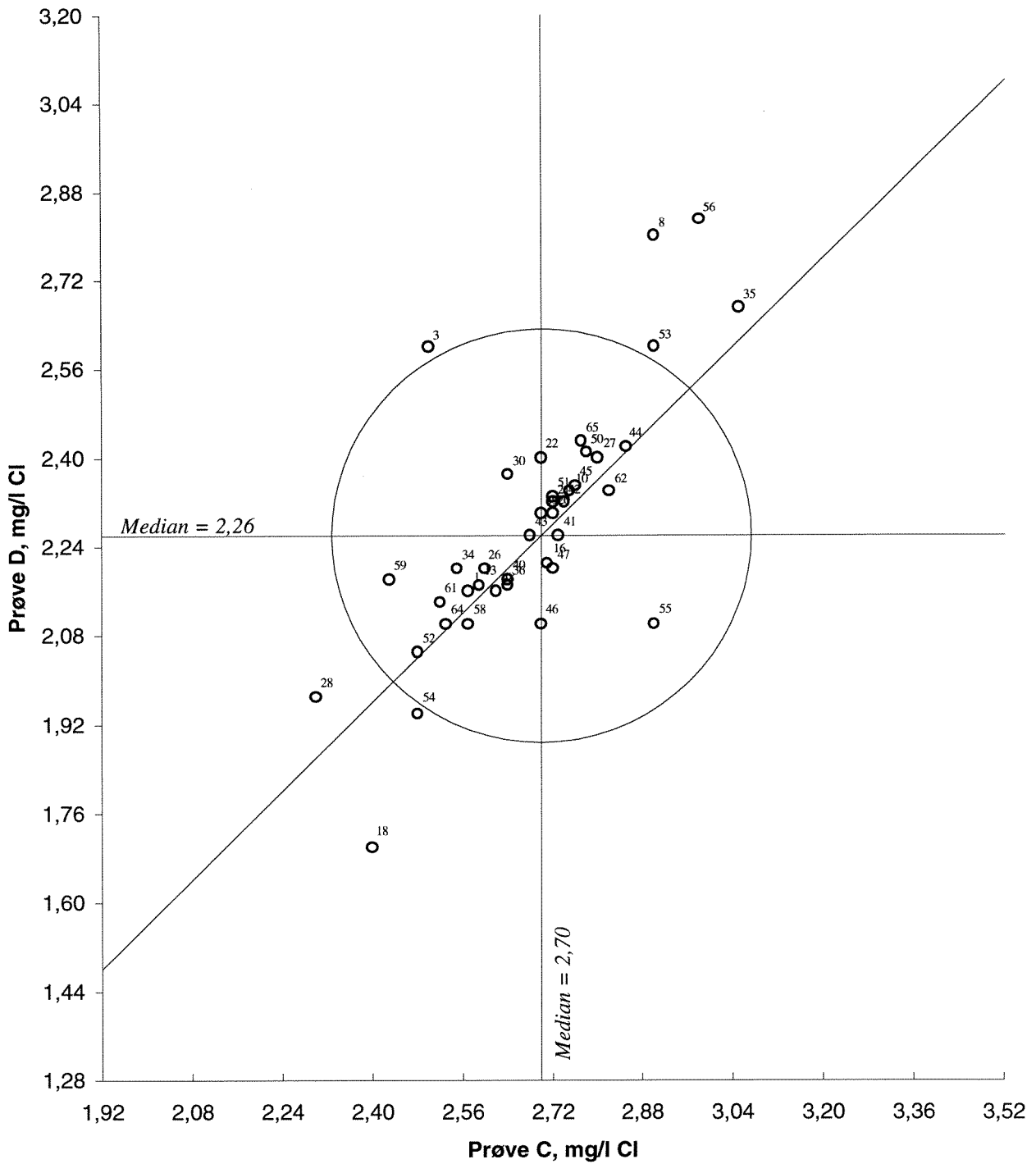
Figur 12. Youdendiagram for klorid, prøvepar CD Akseptansegrensen, angitt med en sirkel, er 15 %
