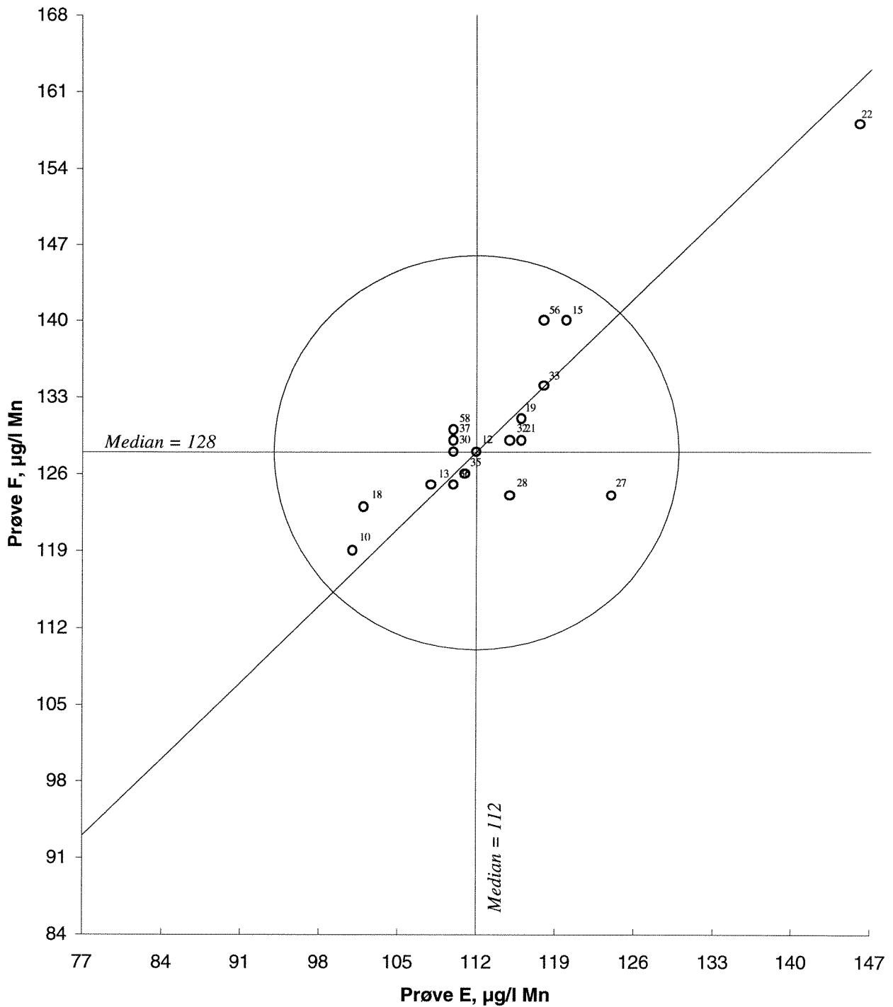
Figur 33. Youdendiagram for mangan, prøvepar EF Akseptansegrensen, angitt med en sirkel, er 15 %
