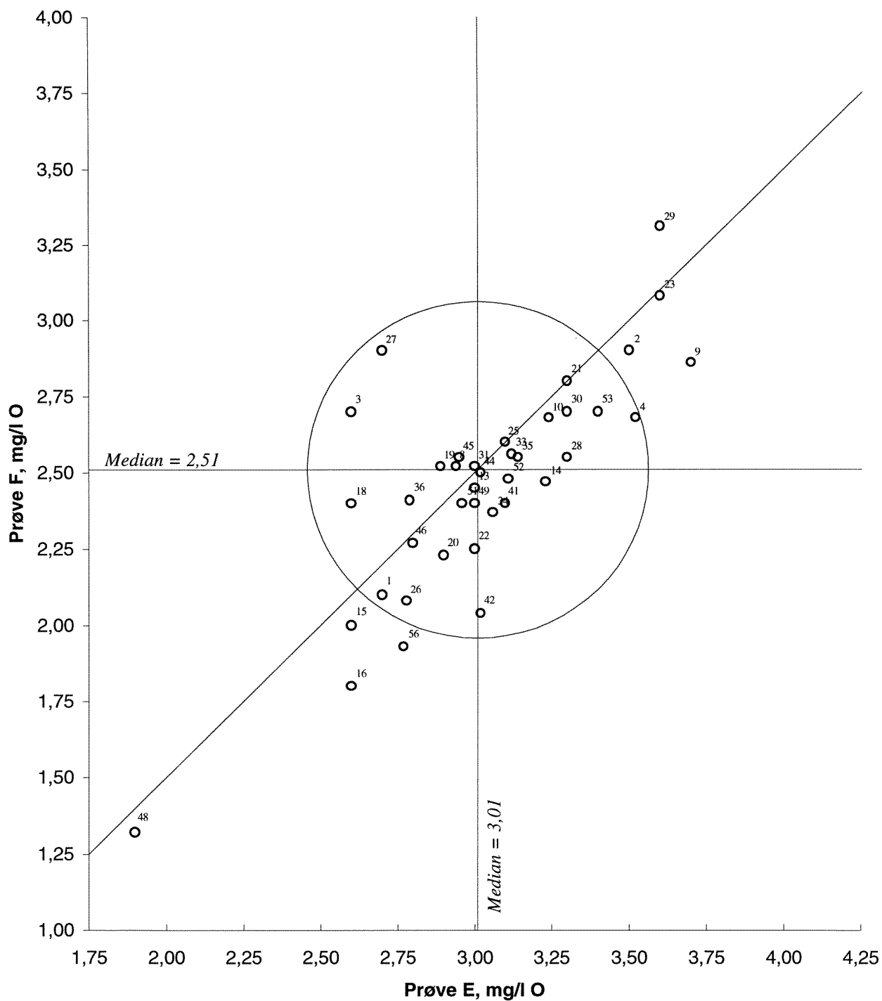
Figur 17. Youdendiagram for kjemisk oksygenforbruk, COD Mn , prøvepar EF Akseptansgrensen, angitt med en sirkel, er 20 %
