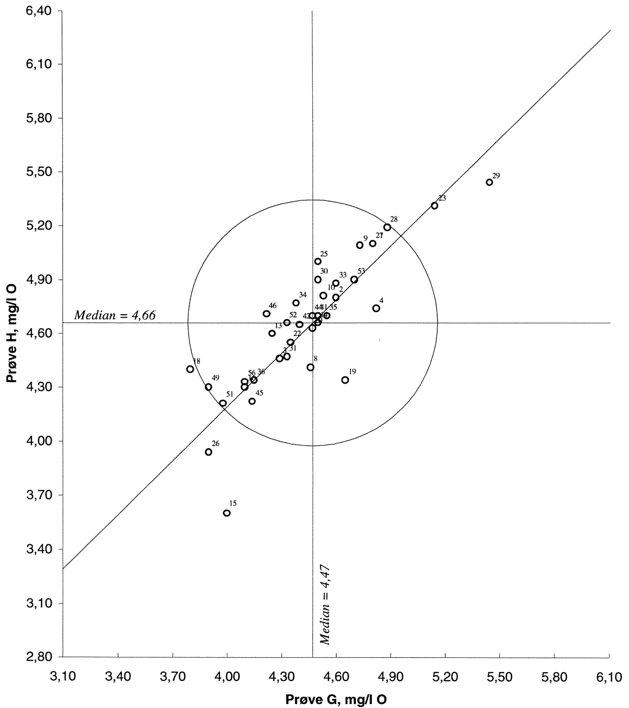
Figur 18. Youtendiagram for kemisk oksygenforbruk, \text{COD}_{\text{Mn}} , prøvepar GH. Akseptansgrensen, angitt med en sirkel, er 15 %
