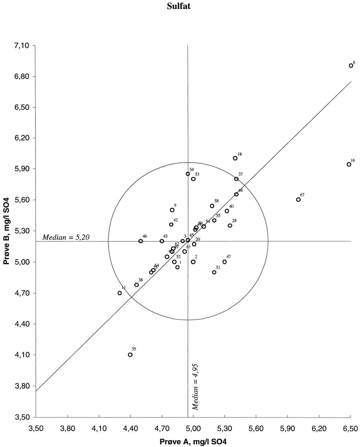
Figur 13. Youdendiagram for sulfat, prøvepar AB Akseptansgrensen, angitt med en sirkel, er 15 %
