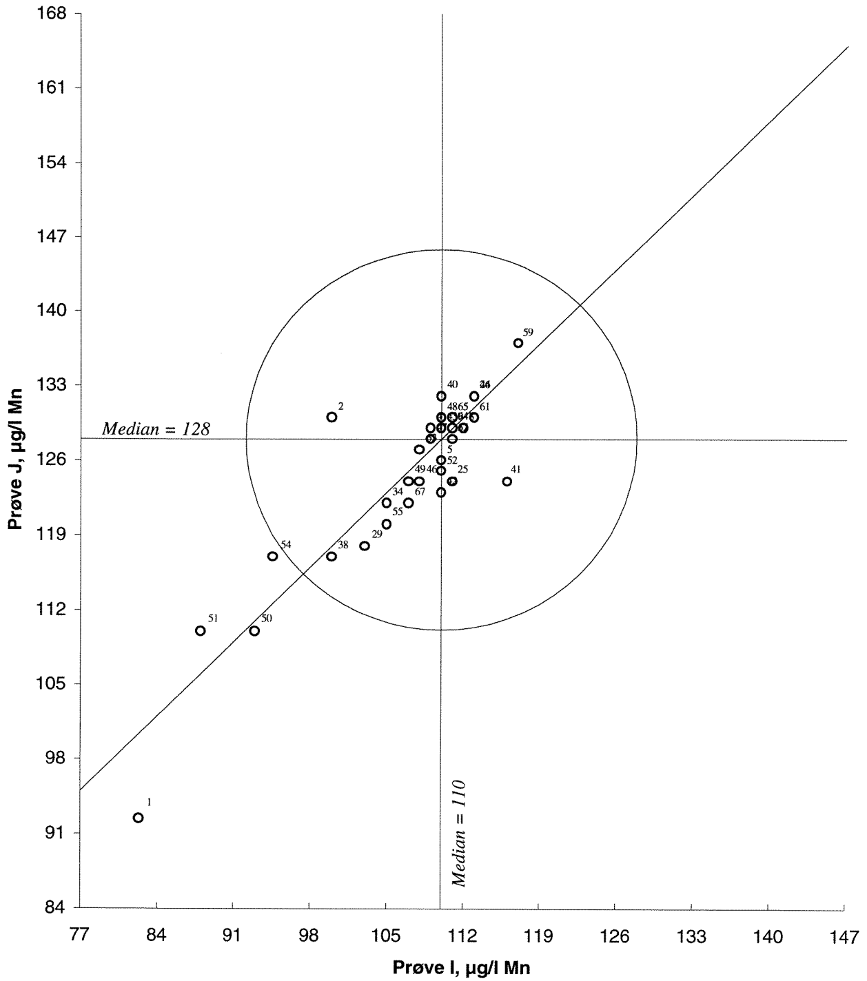
Figur 35. Youndendiagram for mangan, prøvepar IJ Akseptansegrensen, angitt med en sirkel, er 15 %
