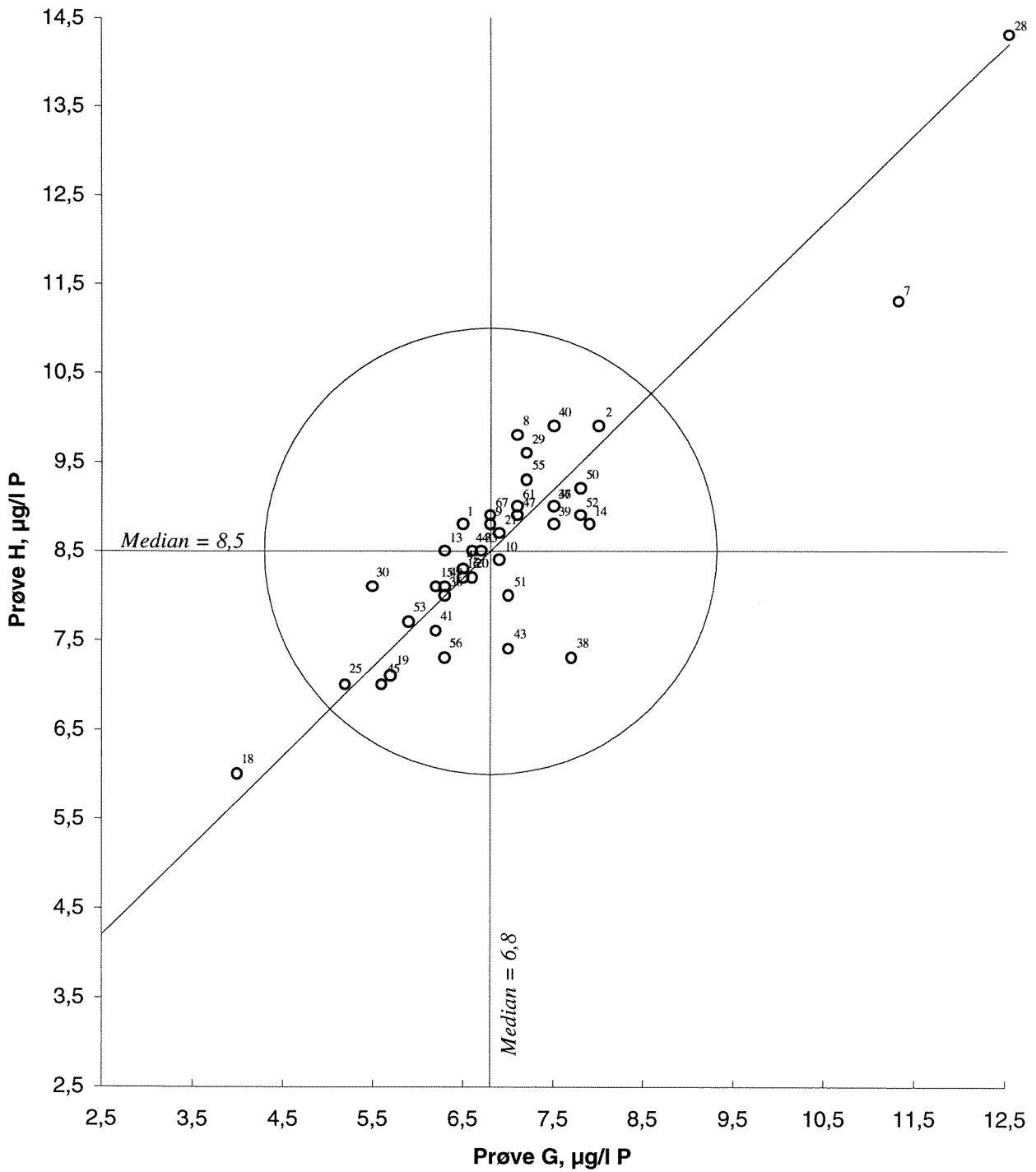
Figur 22. Youndendiagram for totalfosfor, prøvepar GH Akseptansegrensen, angitt med en sirkel, er 2,5 µg/l P
