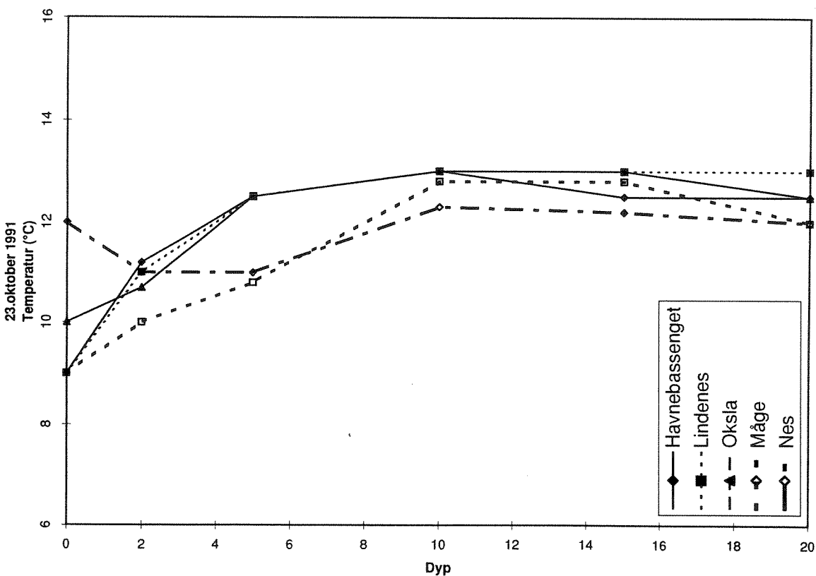
Figur 3.2. Temperaturprofiler i Sør fjorden 23. og 30. oktober 1991.
