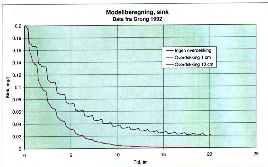
Figur 4. Resultater av modellberegning for sink. Datagrunnlaget er forsøkene fra 1992. Kurvene for 1 og 10 cm overdekking er praktisk talt sammenfallende.
