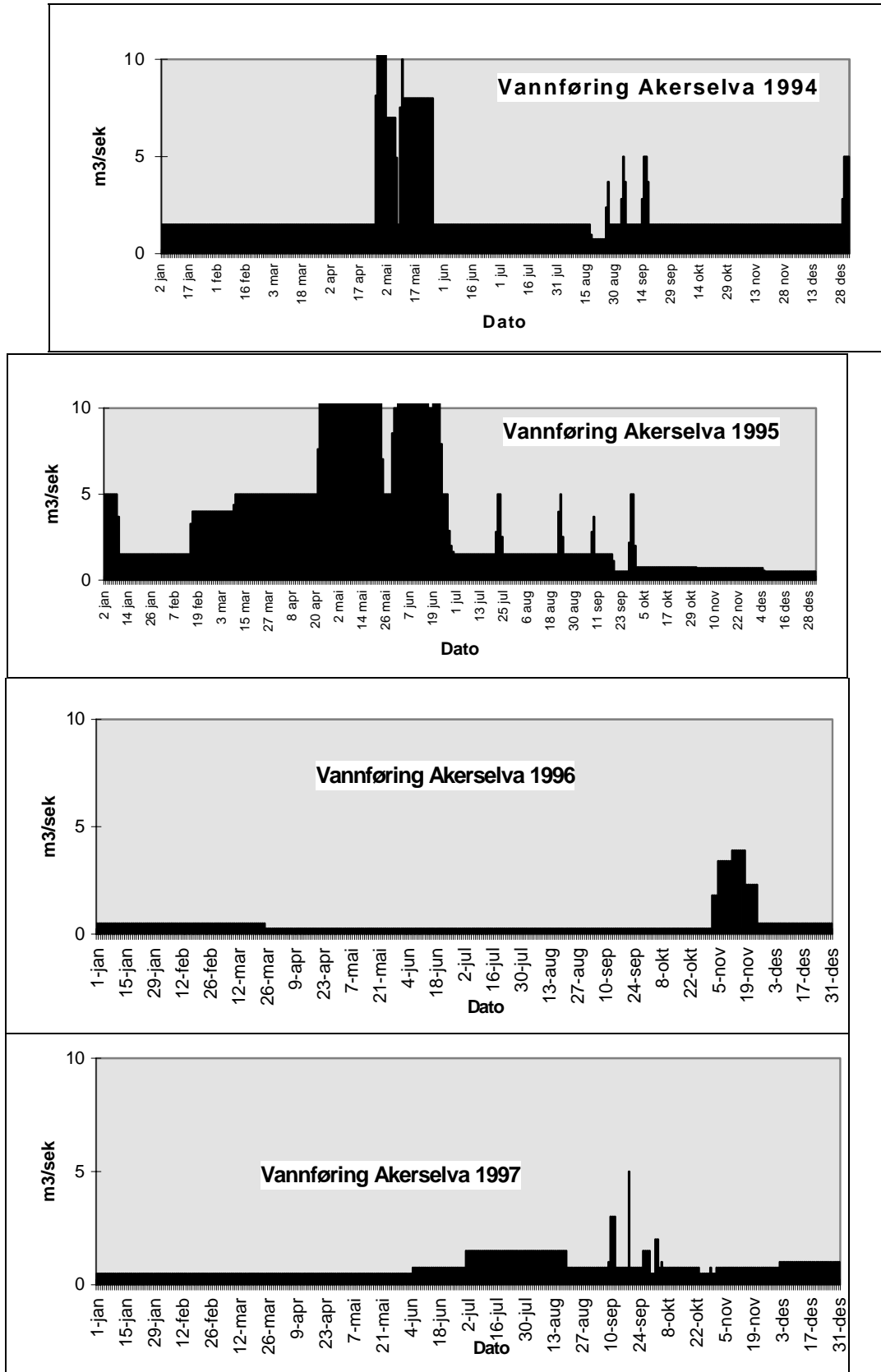
Figur 1. Vannføring øverst i Akerselva i perioden 1/1-90 til 31/12-97. Vannføringer opptil 25 m 3 /sek er registrert, men over 10 m 3 /sek er ikke tegnet inn.
