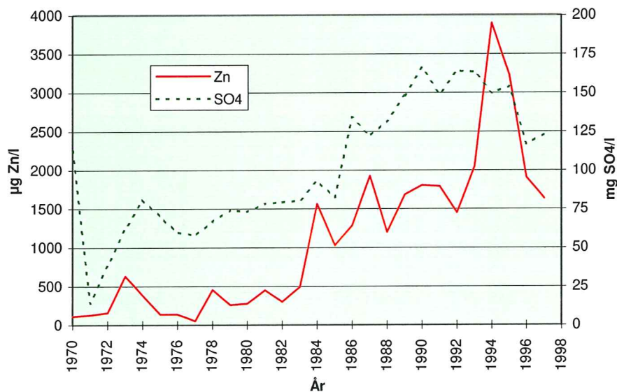
Figur 5. Middelerverdier for sink og sulfat 1970-97. St.2 Gruvevann.
