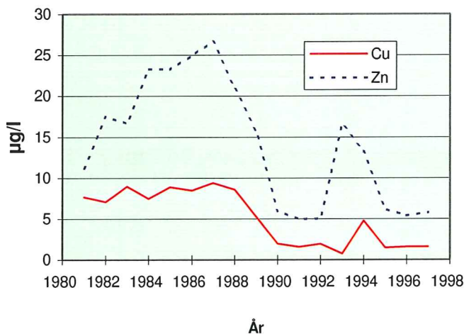
Figur 11. Middelerdier for kobber og sink 1981-97. St. 11 Utløp Vektarbotn.
