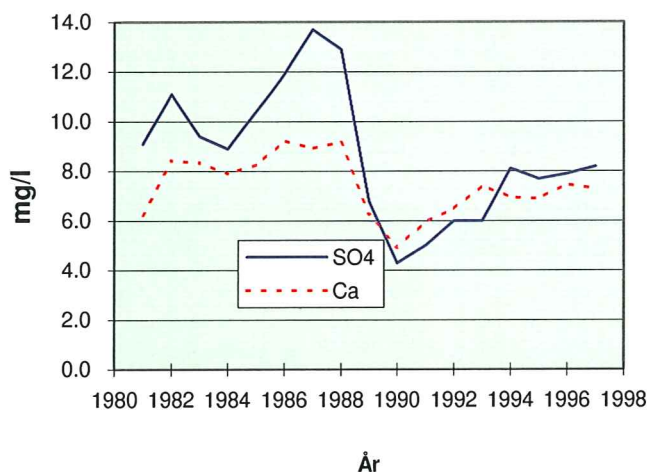
Figur 10. Middelerdier for sulfat og kalsium 1981-97. St. 11 Utløp Vektarbotn.
