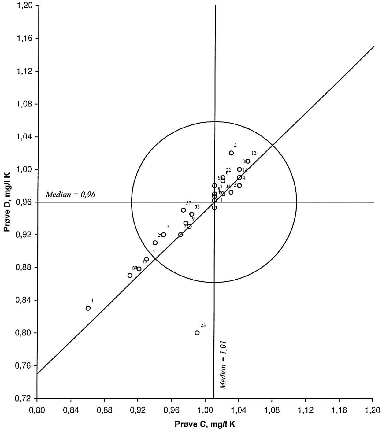
Figur 8. Youdendiagram for kalium, prøvepar CD Akseptansegrensen, angitt med en sirkel, er 10 %
