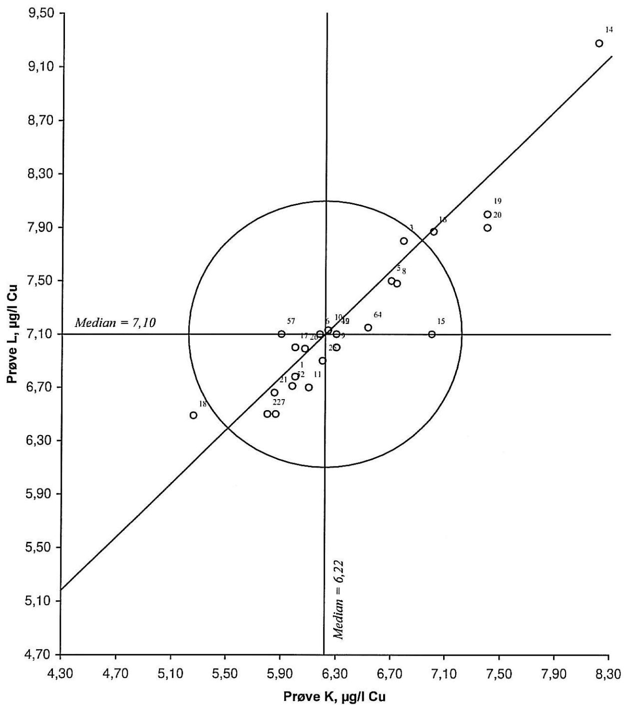
Figur 34. Youtendiagram for kobber, prøvepar KL Akseptansegrensen, angitt med en sirkel, er 1,0 µg/l Cu
