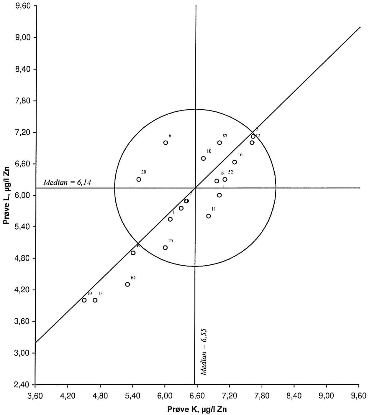
Figur 40. Youdendiagram for sink, prøvepar KL Akseptansegrensen, angitt med en sirkel, er 1,5 µg/l Zn
