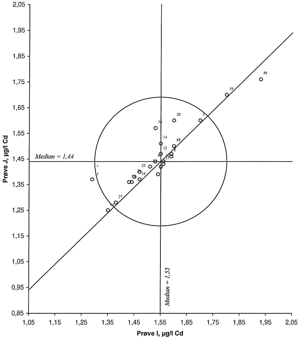
Figur 31. Youtendigram for kadmium, prøvepar IJ Akseptansegrensen, angitt med en sirkel, er 0,25 \mu\text{g/l Cd}
