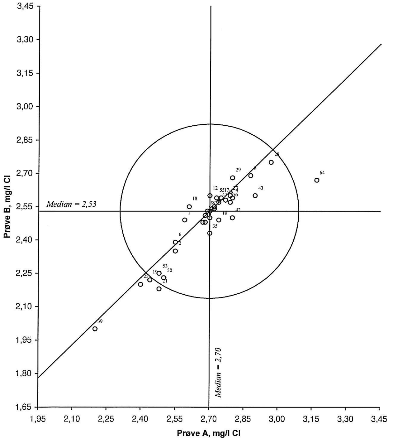
Figur 11. Youdendiagram for klorid, prøvepar AB Akseptansegrensen, angitt med en sirkel, er 15 %
