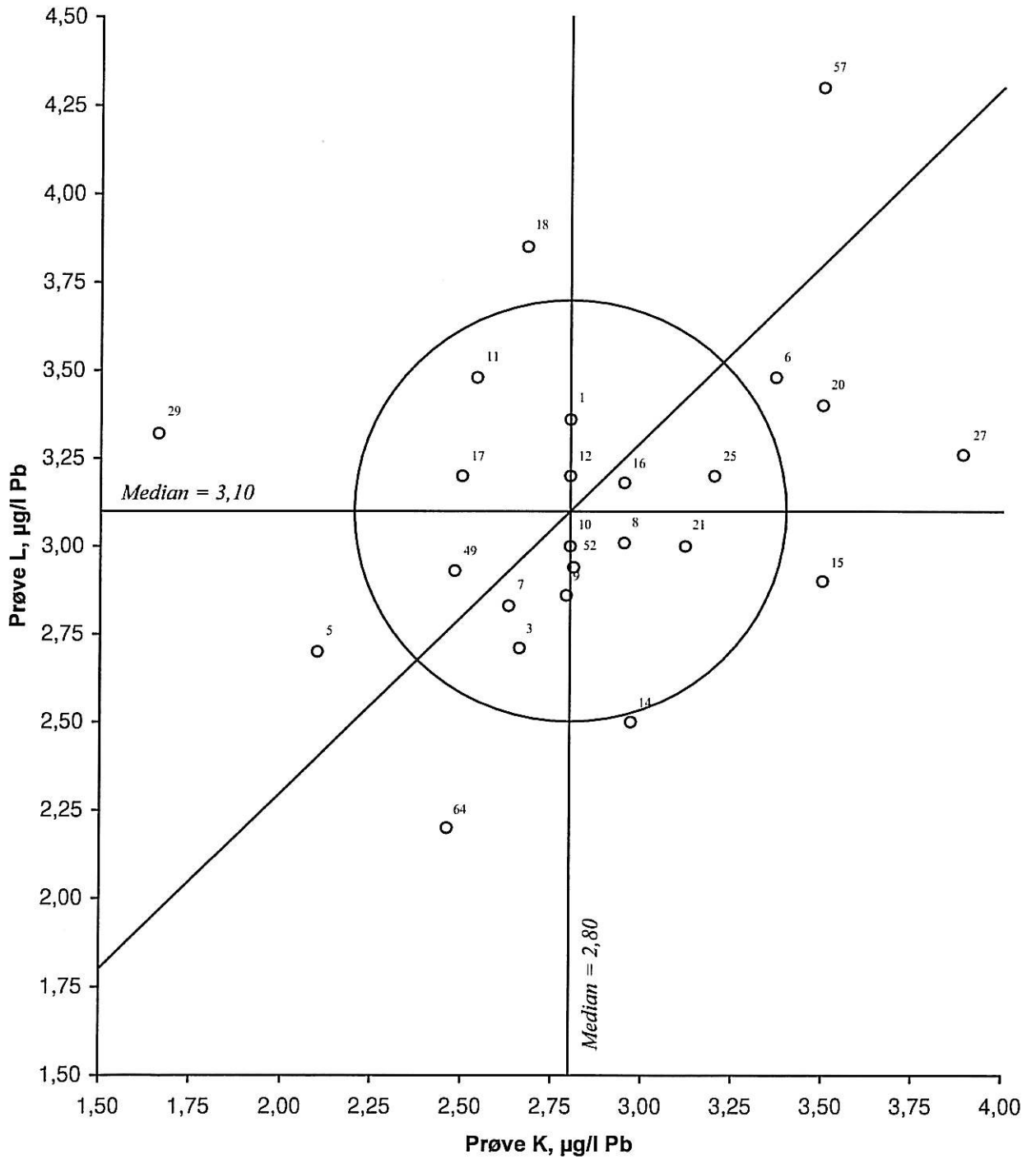
Figur 30. Youdendiagram for bly, prøvepar KL Akseptansegrensen, angitt med en sirkel, er 0,6 µg/l Pb
