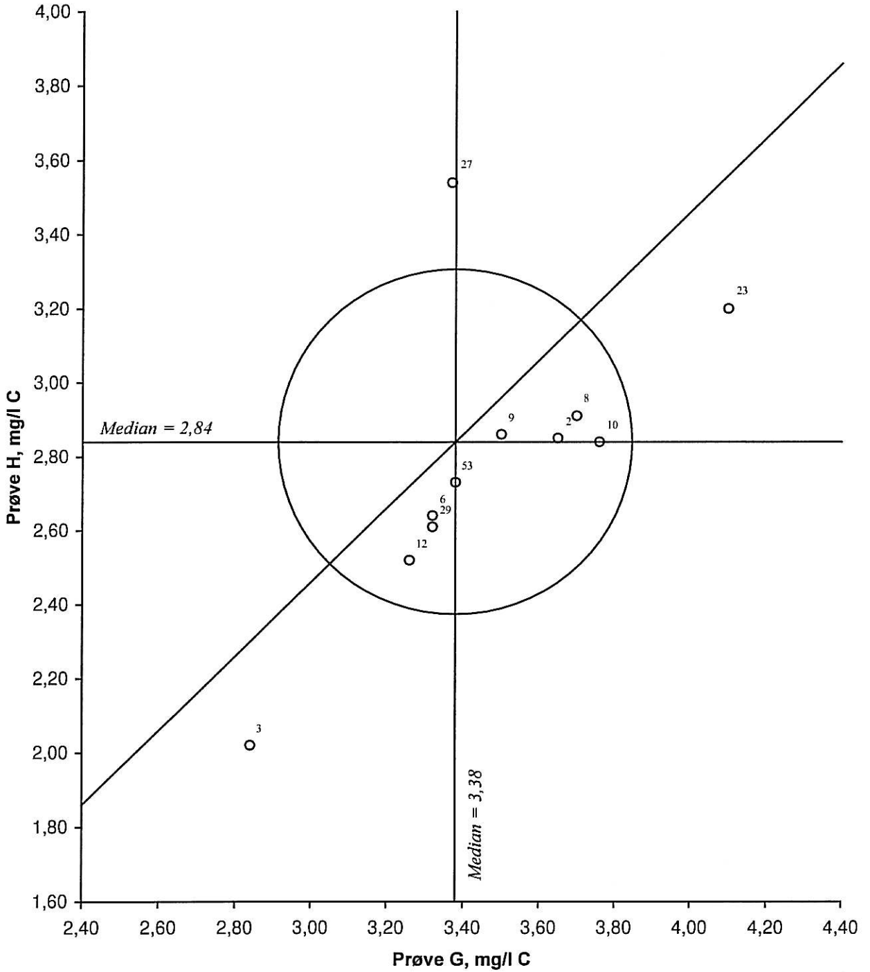
Figur 18. Youdendiagram for totalt organisk karbon, prøvepar GH Akseptansegrensen, angitt med en sirkel, er 15 %
