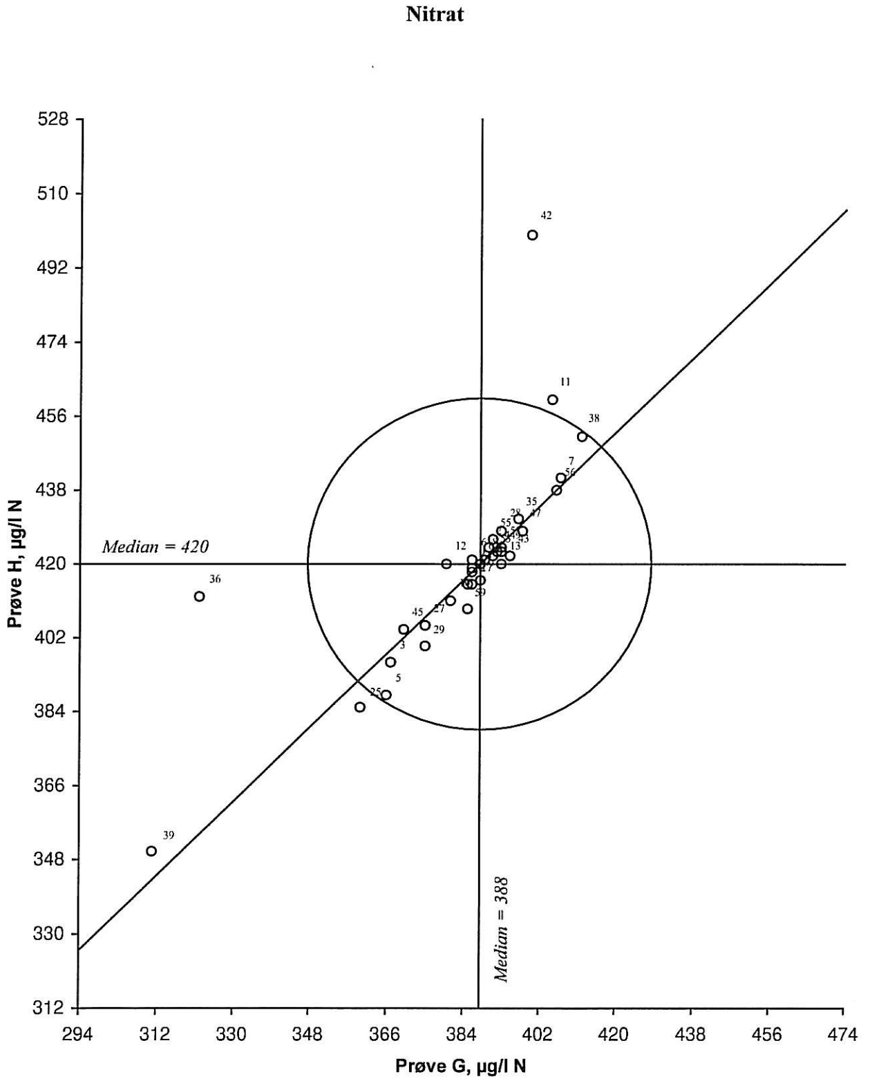
Figur 26. Youdendiagram for nitrat, prøvepar GH Akseptansegrensen, angitt med en sirkel, er 10 %
