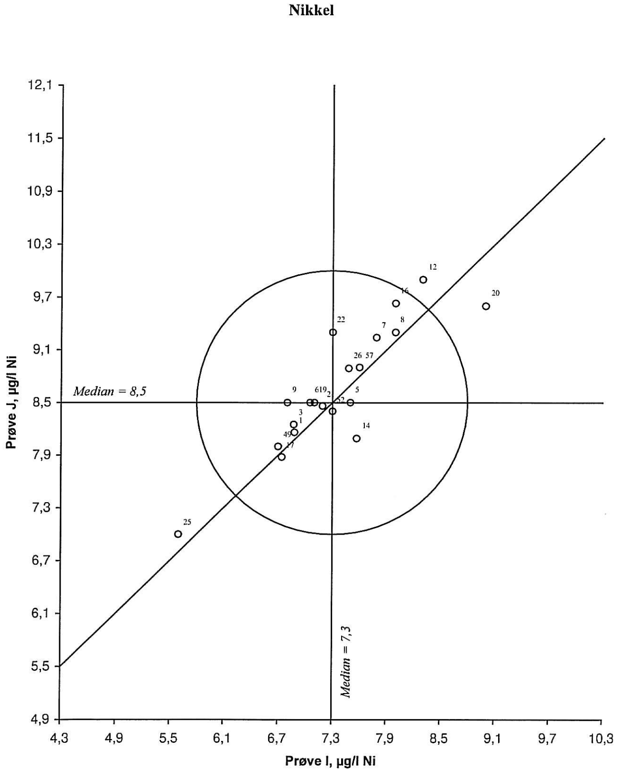
Figur 37. Youdendiagram for nikkel, prøvepar IJ Akseptansegrensen, angitt med en sirkel, er 1,5 µg/l Ni
