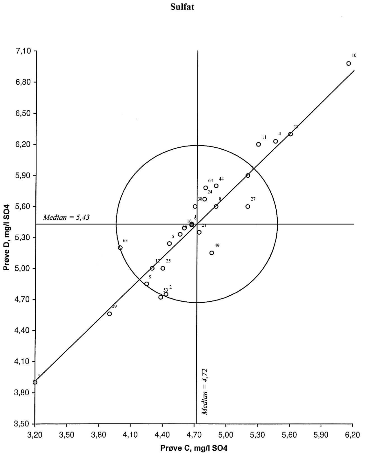
Figur 14. Youtendigram for sulfat, prøvepar CD Akseptansegrensen, angitt med en sirkel, er 15 %
