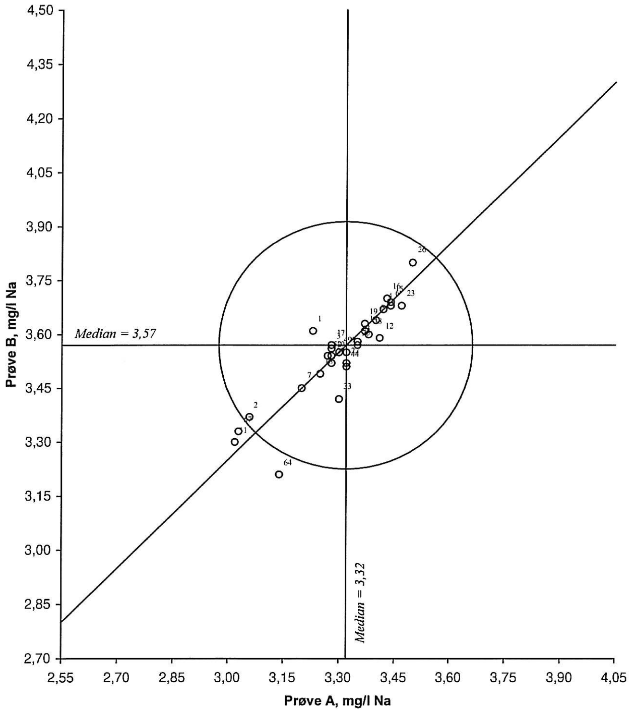
Figur 5. Youdendiagram for natrium, prøvepar AB Akseptansegrensen, angitt med en sirkel, er 10 %
