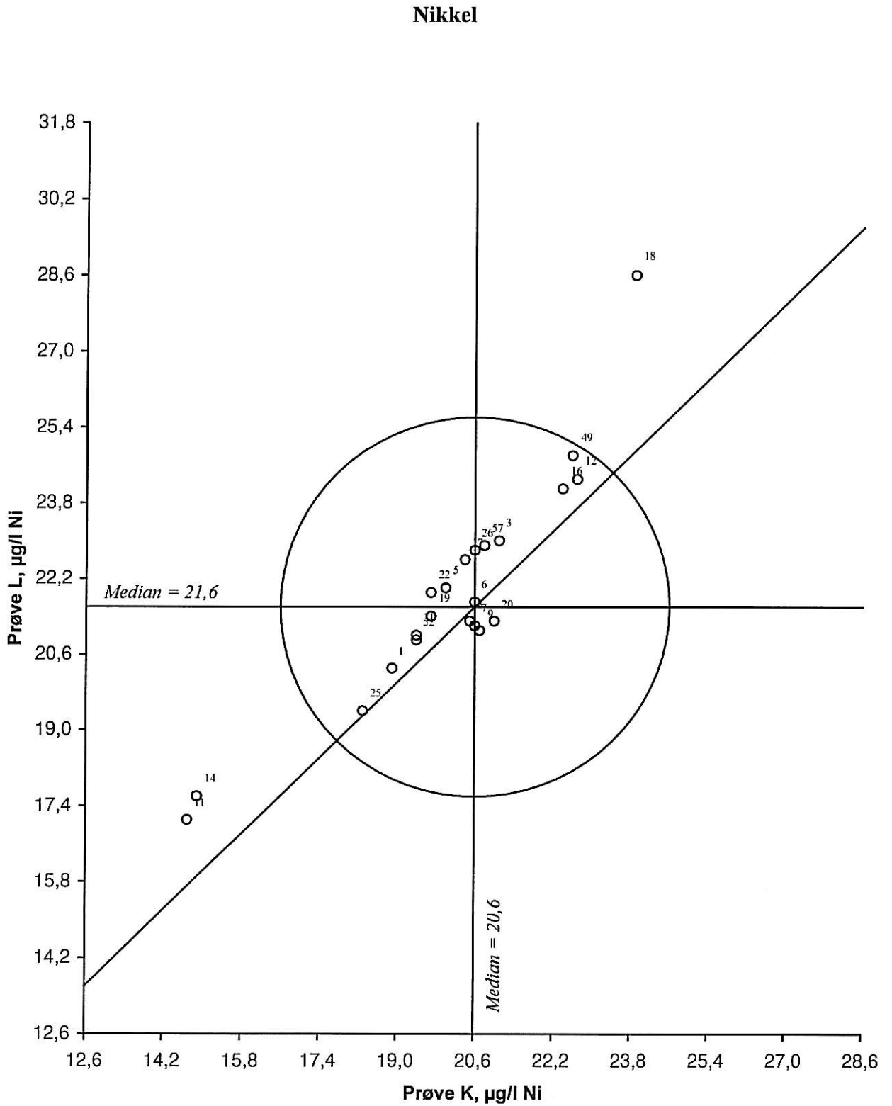
Figur 38. Youtendigram for nikkel, prøvepar KL Akseptansegrensen, angitt med en sirkel, er 4,0 µg/l Ni
