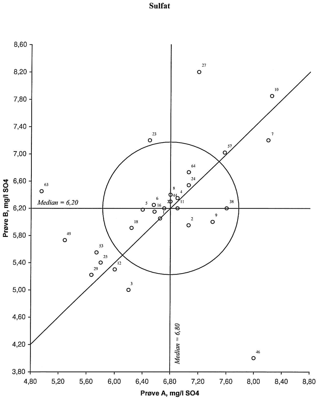
Figur 13. Youdendiagram for sulfat, prøvepar AB Akseptansegrensen, angitt med en sirkel, er 15 %
