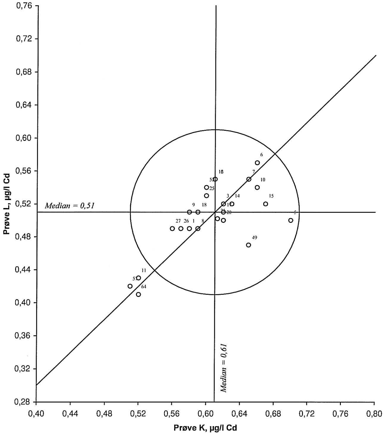
Figur 32. Youdendiagram for kadmium, prøvepar KL Akseptansegrensen, angitt med en sirkel, er 0,10 µg/l Cd
