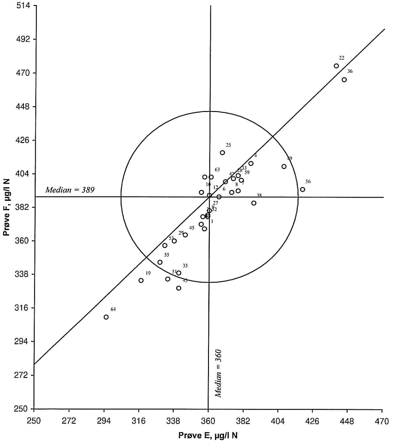
Figur 27. Youtendigram for totalnitrogen, prøvepar EF Akseptansegrensen, angitt med en sirkel, er 15 %
