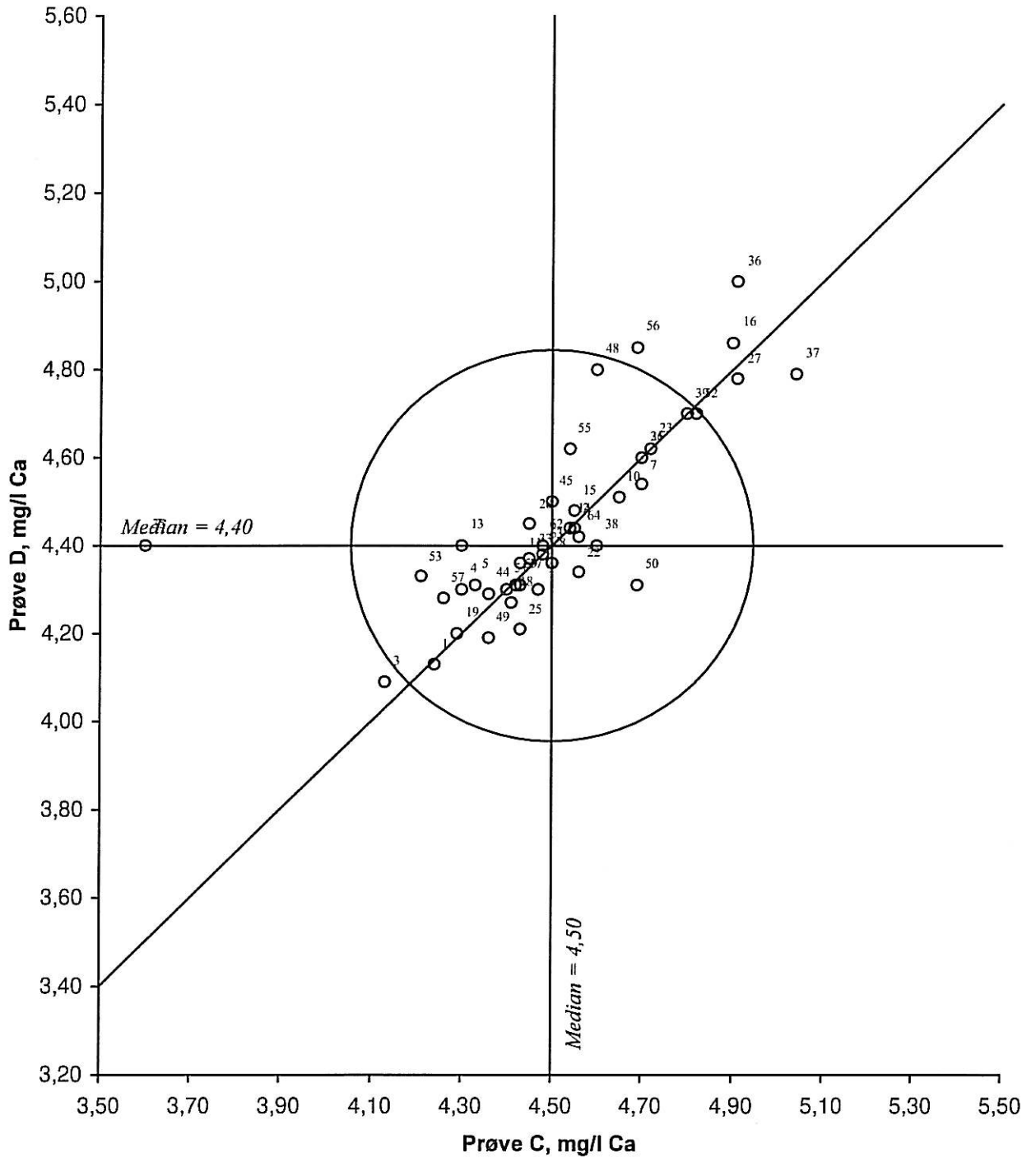
Figur 10. Youtendigram for kalsium, prøvepar CD Akseptansegrensen, angitt med en sirkel, er 10 %
