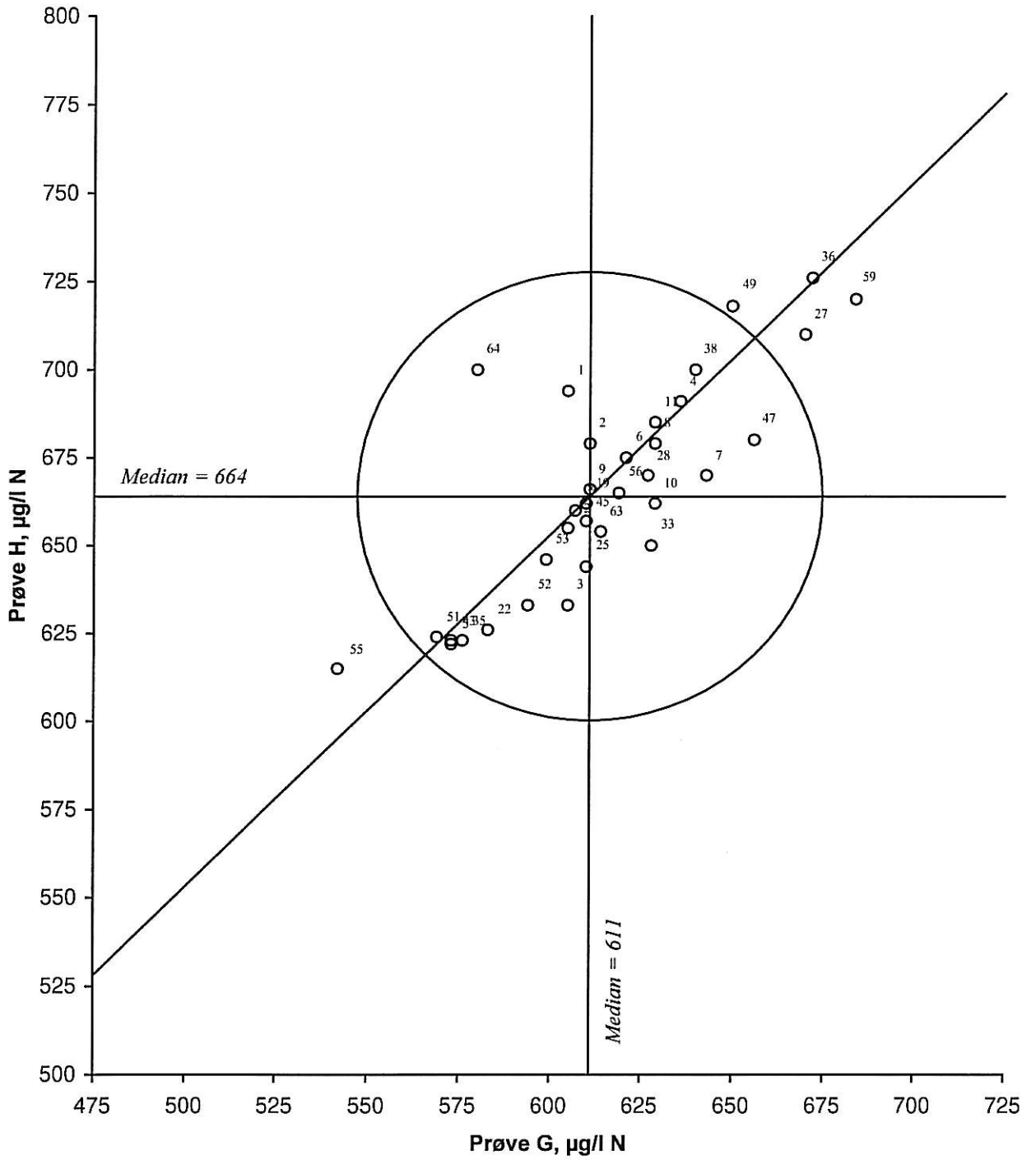
Figur 28. Youndendiagram for totalnitrogen, prøvepar GH Akseptansegrensen, angitt med en sirkel, er 10 %
