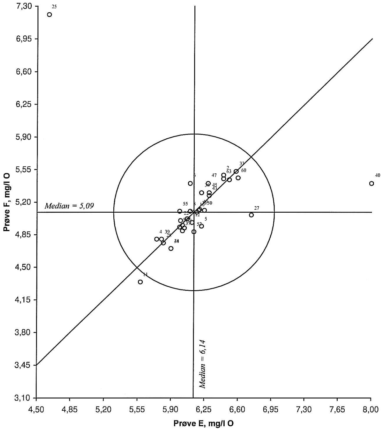
Figur 19. Youtendiagram for kjemisk oksygenforbruk, COD/Mn, prøvepar EF Akseptansegrensen, angitt med en sirkel, er 15 %
