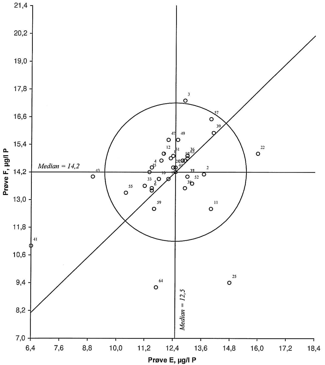
Figur 21. Youdendiagram for totalfosfor, prøvepar EF Akseptansegrensen, angitt med en sirkel, er 3,0 µg/l P
