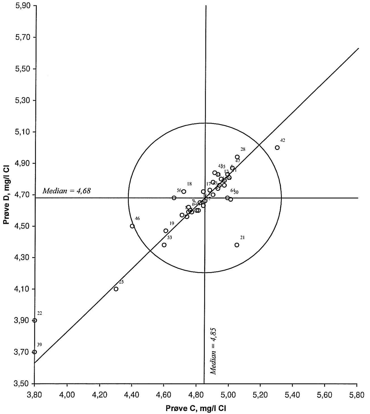
Figur 12. Youdendiagram for klorid, prøvepar CD Akseptansegrensen, angitt med en sirkel, er 10 %
