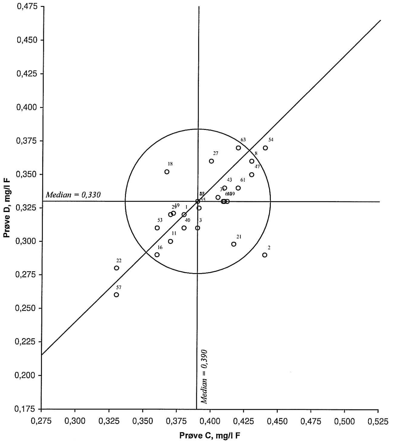
Figur 16. Youndendiagram for fluorid, prøver CD Akseptansegrensen, angitt med en sirkel, er 15 %
