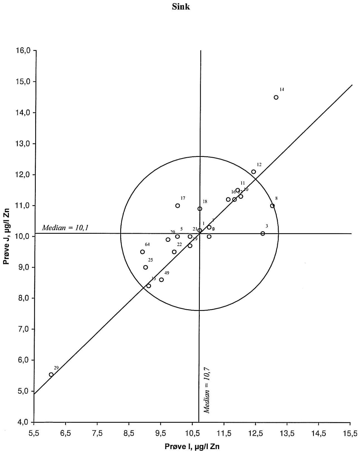
Figur 39. Youtendigram for sink, prøvepar IJ Akseptansegrensen, angitt med en sirkel, er 2,5 µg/l Zn
