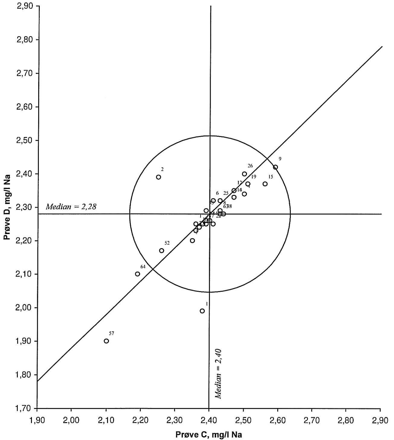
Figur 6. Youdendiagram for natrium, prøvepar CD Akseptansegrensen, angitt med en sirkel, er 10 %
