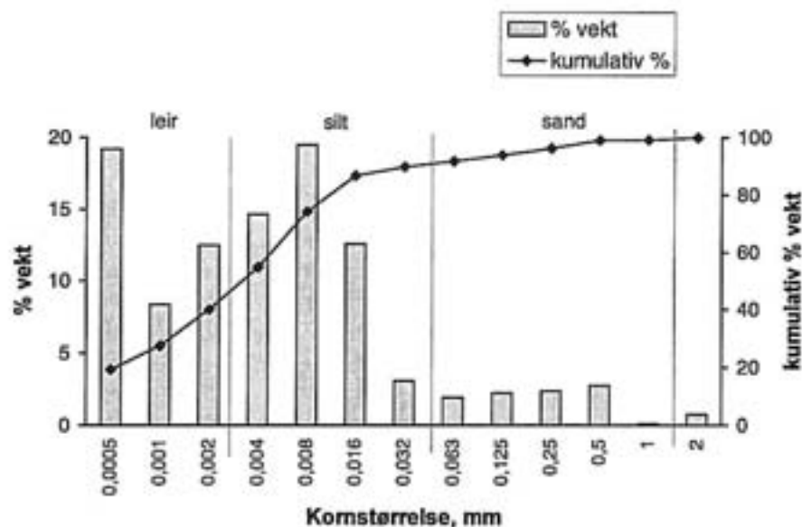
Figur 7. Partikkelfordeling i overflatesediment fra stasjon TVE 10 i nærsonen til oppdrettsanlegget i Oksefjorden.
