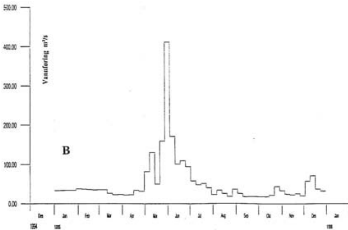
Figur 4. B : Karakteristiske 7-døgns midler for vannføringen i Orkla ved Syrstad i 1995.
