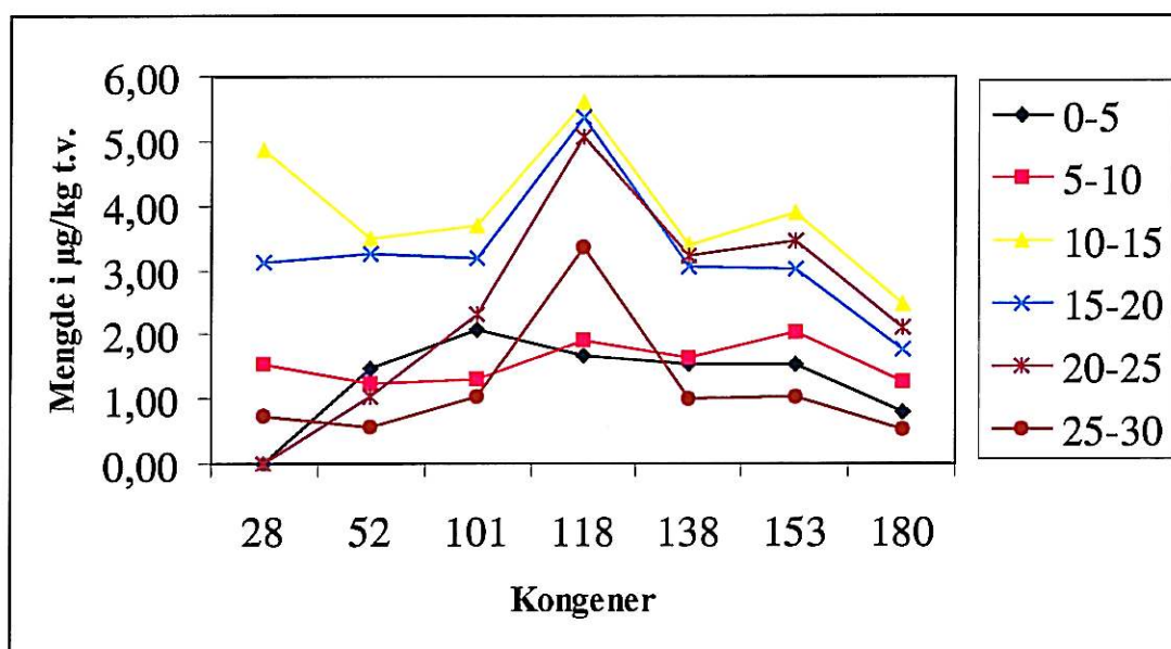
Figur 13. Fordeling av 7-PCB kongener i kjerneprøver fra Drammensfjorden, stasjon D2
