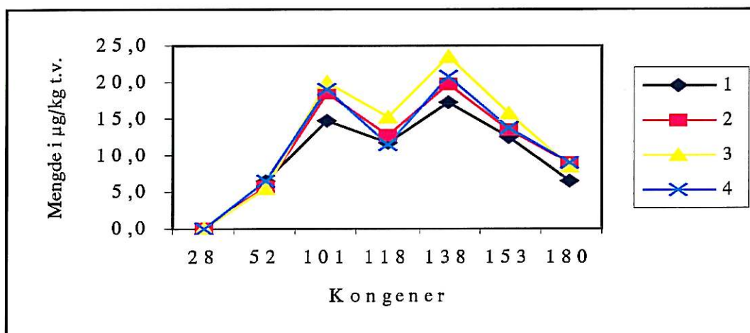
Figur 12. Fordeling av 7-PCB kongener i prøver fra Oslofjorden, stasjon O-2, paralell 1-4
