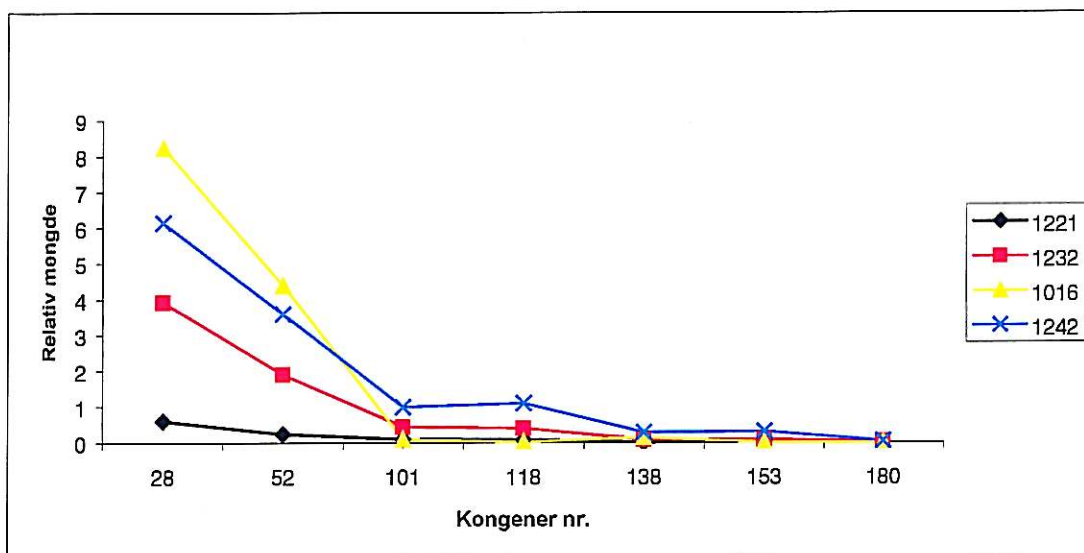
Figur 7. Sammensetning av 7-PCB kongener (PCB nr. 28, 52, 101, 118, 138, 153 og 180) i forskjellige Aroclor-blandingene 1221, 1232, 1016 og 1242.
