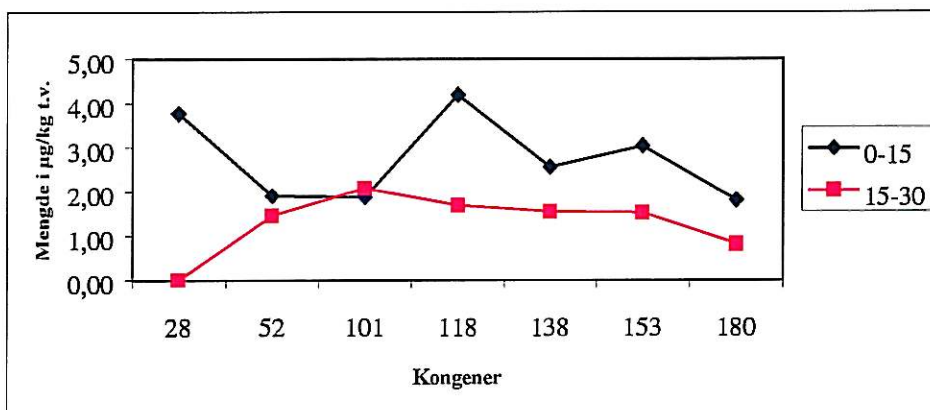
Figur 14. Fordeling av 7-PCB kongener i kjerneprøver fra Drammensfjorden, stasjon D3
