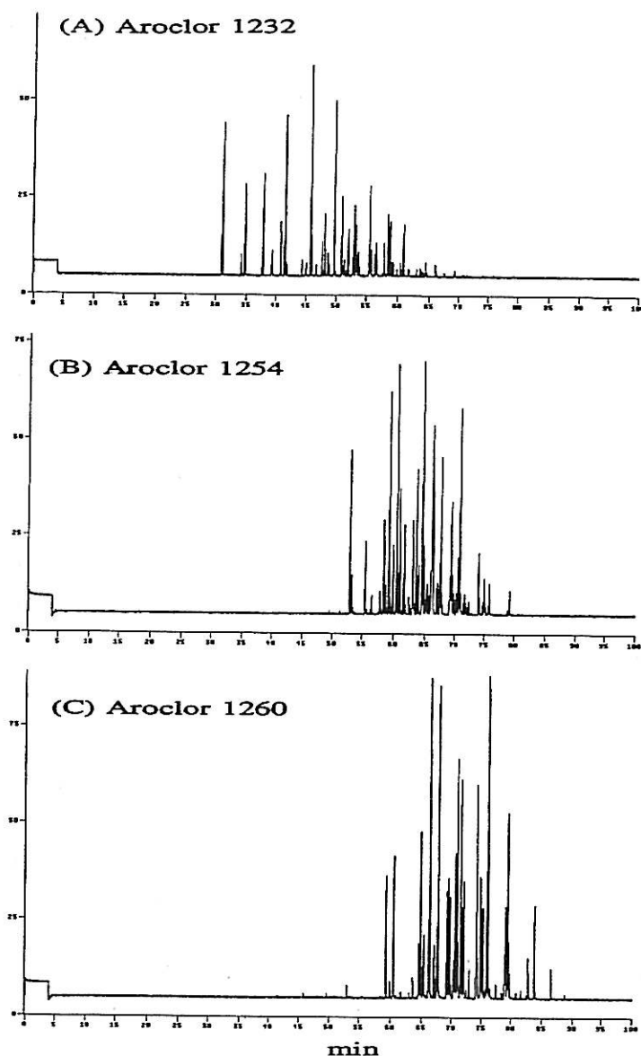
Figur 5. Klor-selektivte GC-AED kromatogrammer av tekniske blandinger med kloreringsgrad på h.h.v. 32%, 54% og 60%.
