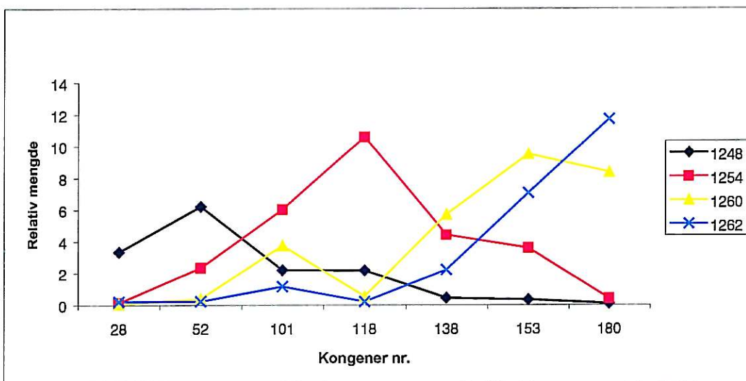
Figur 8. Sammensetning av 7-PCB kongener (PCB nr. 28, 52, 101, 118, 138, 153 og 180) i forskjellige Aroclor-blandingene 1248, 125,1260 og 1262.
